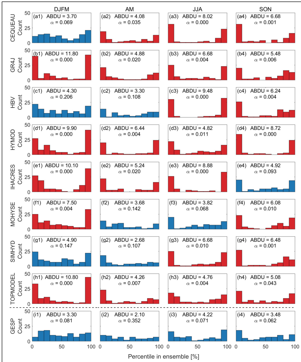
Figure 3.3 Diagrammes de Talagrand représentant le rang (en percentiles) occupé par les débits observés dans les ESPs des huit modèles hydrologiques différents après avoir effectué le DA et le QM sur le bassin versant PD. Les diagrammes en bleu (rouge) indiquent que l'hypothèse d'uniformité n'est pas rejetée (rejetée) par le test K-S ( \alpha = 0,05 )
