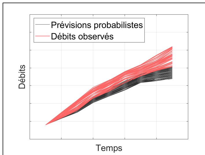
Figure 1.3 Exemple d'un ensemble hydrologique prévisionnel systématiquement biaisé négativement. Les observations ne sont pas incluses dans l'ensemble
