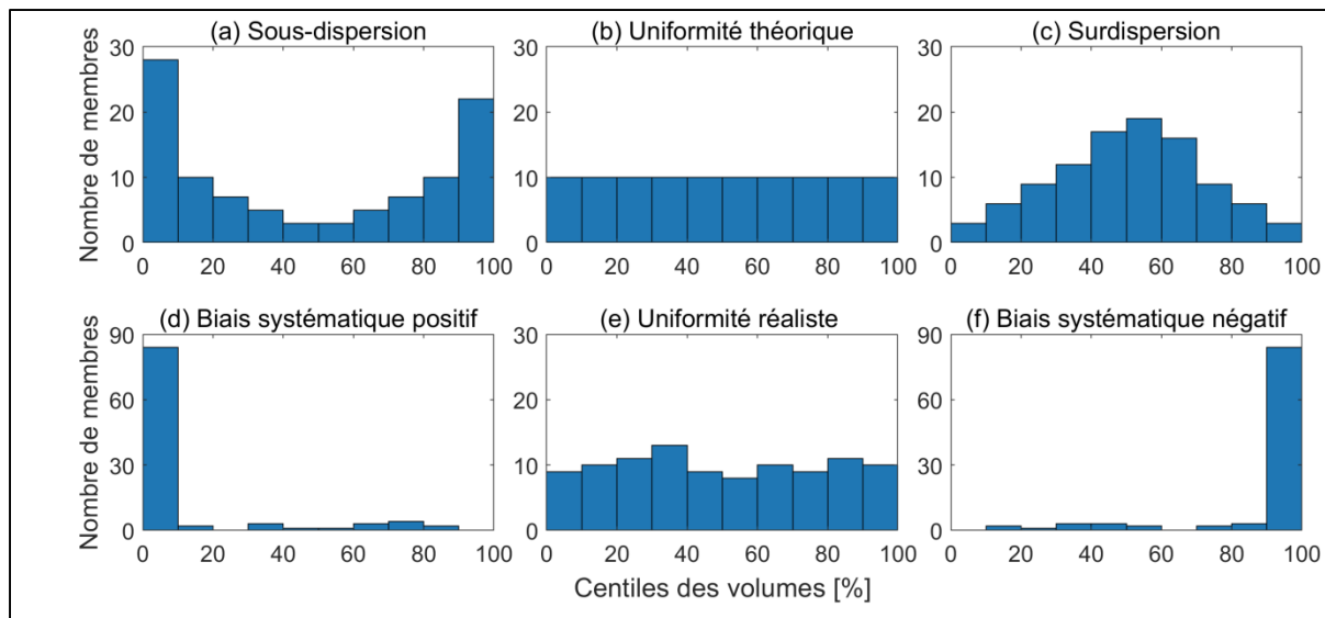
Figure 1.2 Exemples de dispersion d'un ensemble de 100 membres sur des diagrammes de Talagrand. Le « Nombre de membres » en ordonnée du diagramme représente la fréquence des observations, c'est-à-dire le nombre de fois où l'observation se situe dans une des 10 classes en abscisse du diagramme de Talagrand
