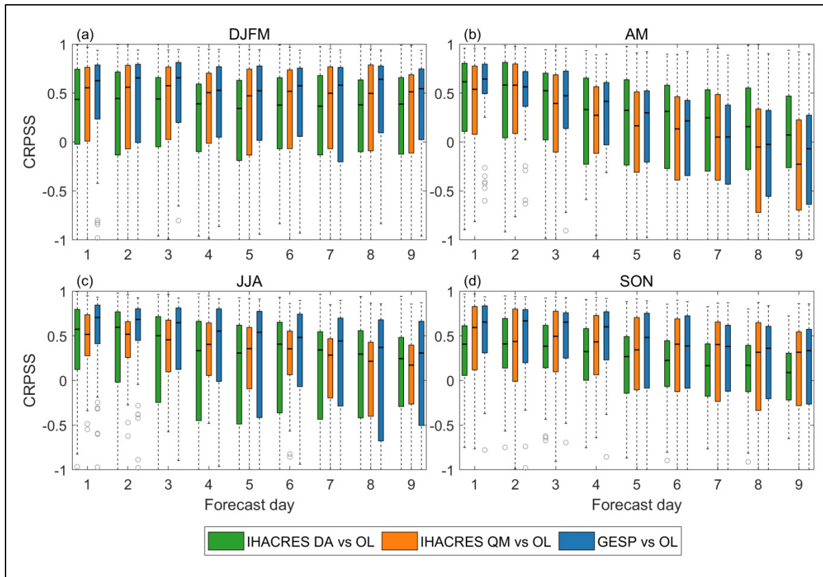
Figure-A II-4 Boîtes à moustaches des valeurs CRPSS des membres de l'ensemble hydrologique du modèle IHACRES et de l'ensemble multi-modèles (GESP) sur le bassin versant CS. Un CRPSS supérieur à zéro indique une amélioration de la précision globale des prévisions par rapport aux simulations de référence (OL) d'IHACRES. Les membres dont les valeurs du CRPSS sont inférieures à -1 sont considérés comme très mauvais et ne sont pas indiqués afin d'éviter de surcharger le graphique
