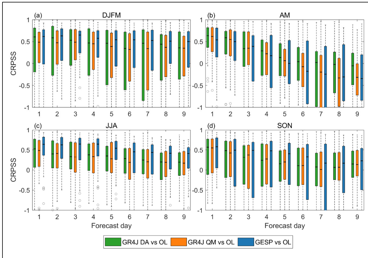
Figure-A II-2 Boîtes à moustaches des valeurs CRPSS des membres de l'ensemble hydrologique du modèle GR4J et de l'ensemble multi-modèles (GESP) sur le bassin versant CS. Un CRPSS supérieur à zéro indique une amélioration de la précision globale des prévisions par rapport aux simulations de référence (OL) de GR4J. Les membres dont les valeurs du CRPSS sont inférieures à -1 sont considérés comme très mauvais et ne sont pas indiqués afin d'éviter de surcharger le graphique
