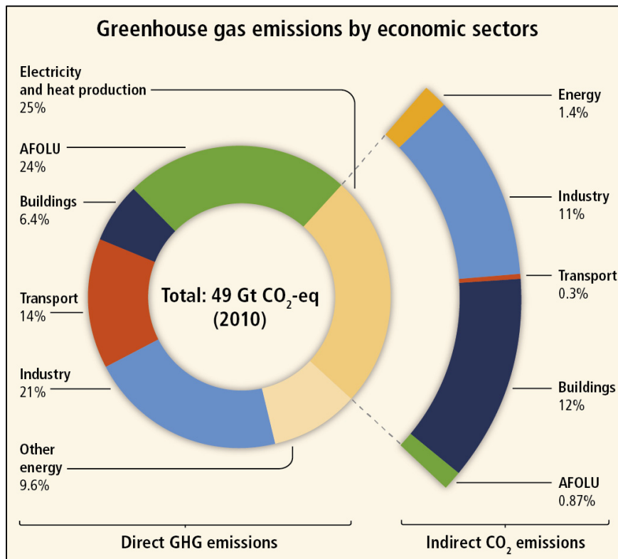
Figure 0.1 Émissions de GES d'origine anthropique par secteurs d'activité en 2010. Le secteur de l'énergie comprend la production d'électricité, de chaleur et des autres énergies. Les secteurs placés dans la section « Indirect CO 2 emissions » représentent les utilisateurs de l'énergie électrique et de la production de chaleur. Le terme AFOLU correspond à « agriculture, forestry and other land use » Tirée du rapport synthèse AR5 (p.47) IPCC et al. (2014)
