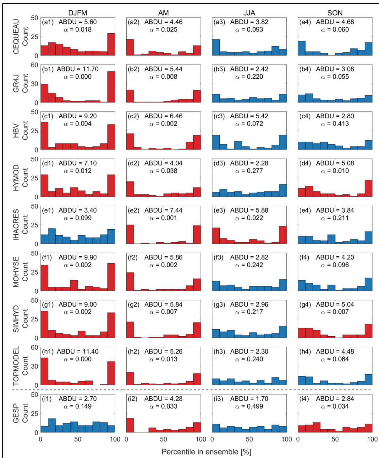
Figure-A I-2 Diagrammes de Talagrand représentant le rang (en percentiles) occupé par les débits observés dans les ESPs des huit modèles hydrologiques différents après avoir effectué le DA et le QM sur le bassin versant CD. Les diagrammes en bleu (rouge) indiquent que l'hypothèse d'uniformité n'est pas rejetée (rejetée) par le test K-S ( \alpha = 0,05 )
