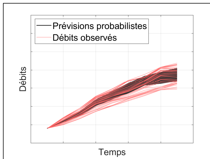
Figure 1.1 Exemple d'un ensemble hydrologique prévisionnel sous-dispersé. La dispersion de l'ensemble n'est pas assez grande pour inclure tous les débits observés
