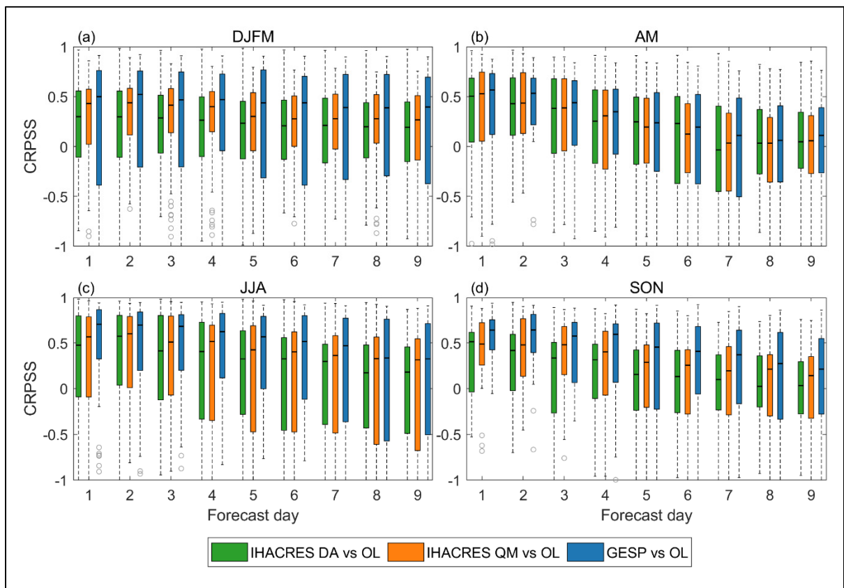
Figure 3.2 Boîtes à moustaches des valeurs CRPSS des membres de l'ensemble hydrologique du modèle IHACRES et de l'ensemble multi-modèles (GESP) sur le bassin versant LSJ. Un CRPSS supérieur à zéro indique une amélioration de la précision globale des prévisions par rapport aux simulations de référence (OL) d'IHACRES. Les membres dont les valeurs du CRPSS sont inférieures à -1 sont considérés comme très mauvais et ne sont pas indiqués afin d'éviter de surcharger le graphique
