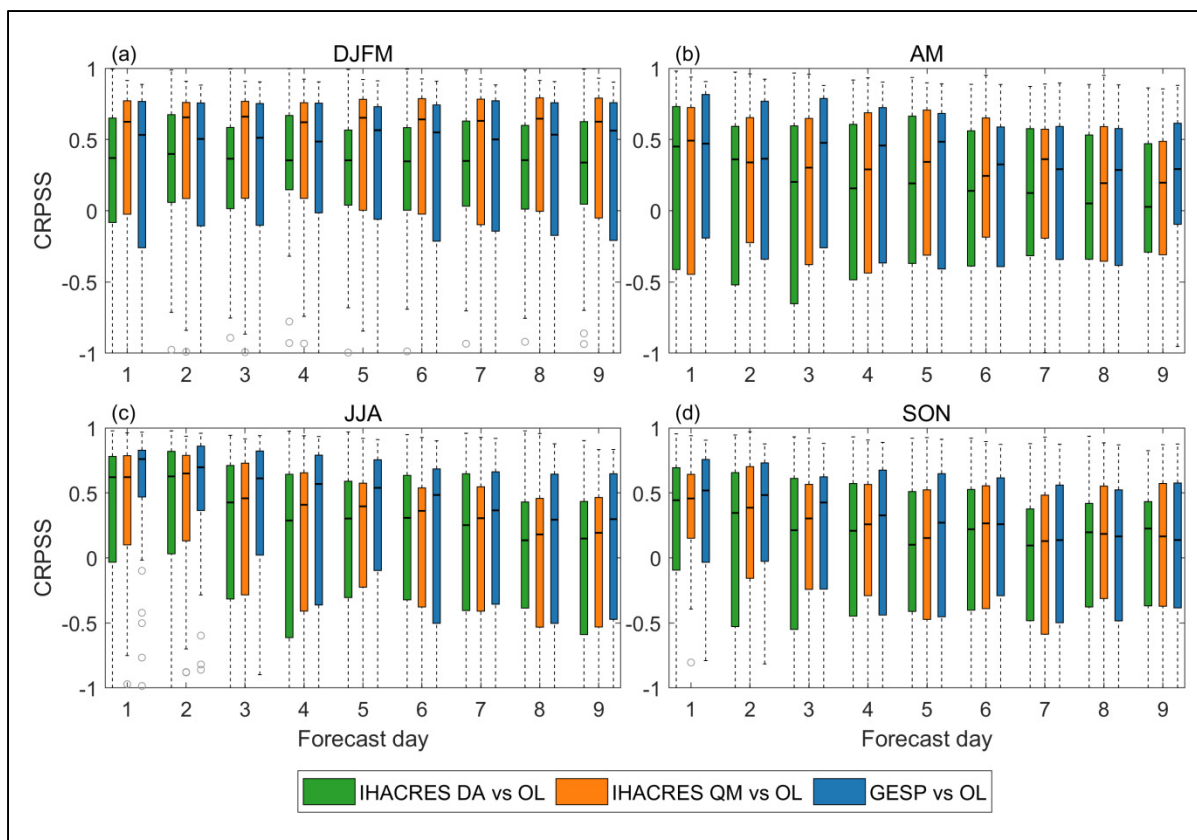
Figure-A II-3 Boîtes à moustaches des valeurs CRPSS des membres de l'ensemble hydrologique du modèle IHACRES et de l'ensemble multi-modèles (GESP) sur le bassin versant LM. Un CRPSS supérieur à zéro indique une amélioration de la précision globale des prévisions par rapport aux simulations de référence (OL) d'IHACRES. Les membres dont les valeurs du CRPSS sont inférieures à -1 sont considérés comme très mauvais et ne sont pas indiqués afin d'éviter de surcharger le graphique
