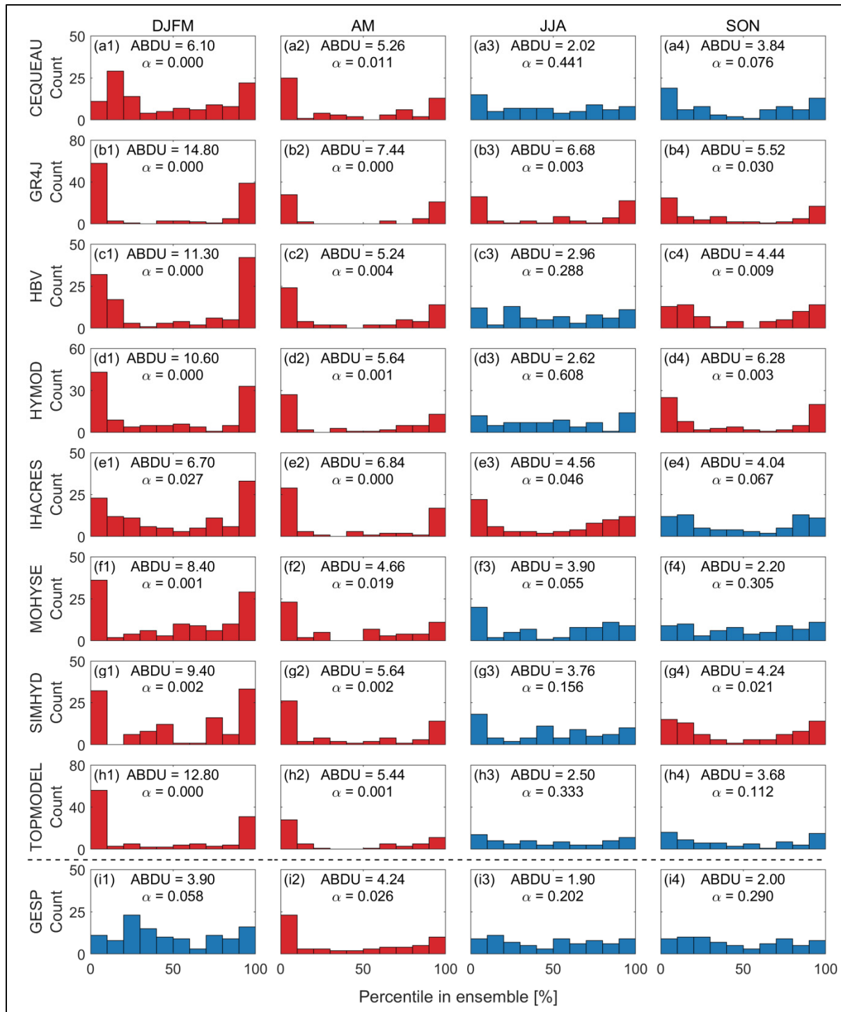
Figure-A I-3 Diagrammes de Talagrand représentant le rang (en percentiles) occupé par les débits observés dans les ESPs des huit modèles hydrologiques différents après avoir effectué le DA et le QM sur le bassin versant CS. Les diagrammes en bleu (rouge) indiquent que l'hypothèse d'uniformité n'est pas rejetée (rejetée) par le test K-S ( \alpha = 0,05 )
