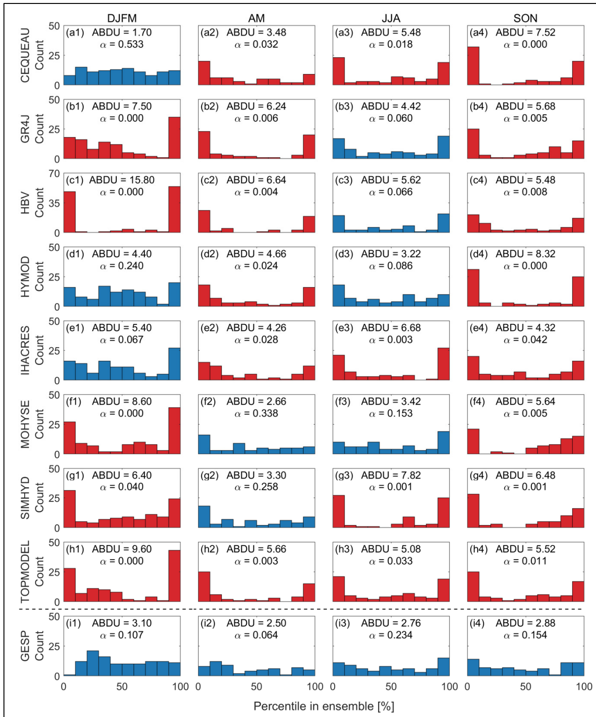
Figure-A I-1 Diagrammes de Talagrand représentant le rang (en percentiles) occupé par les débits observés dans les ESPs des huit modèles hydrologiques différents après avoir effectué le DA et le QM sur le bassin versant LM. Les diagrammes en bleu (rouge) indiquent que l'hypothèse d'uniformité n'est pas rejetée (rejetée) par le test K-S ( \alpha = 0,05 )
