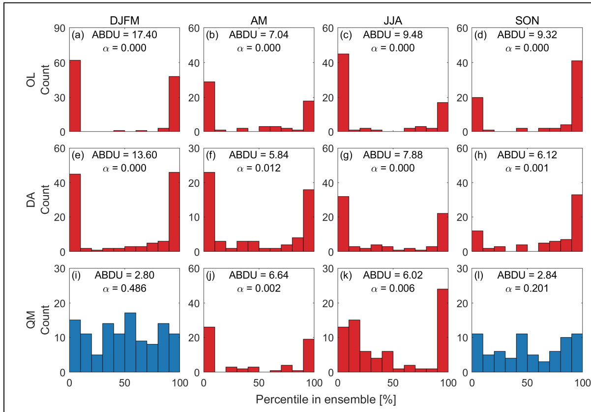
Figure 3.1 Diagrammes de Talagrand représentant le rang (en percentiles) occupé par les débits observés dans l'ensemble des prévisions hydrologiques à l'aide du modèle IHACRES sur le bassin versant LSJ. "OL" fait référence à la simulation de référence. "DA" réfère aux membres de validation des 1250 membres de l'ensemble après avoir effectué l'assimilation des données et "QM" réfère aux mêmes membres après avoir effectué l'assimilation des données et le post-traitement avec la correction par quantiles. Les diagrammes en bleu (rouge) indiquent que l'hypothèse d'uniformité n'est pas rejetée (rejetée) par le test K-S ( \alpha = 0,05 )
