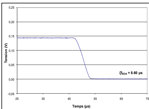
Figure 2.31 Tracé descente à 10µs (cas B).
