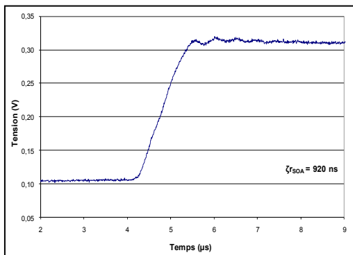
Figure 2.21 Tracé montée à 1µs (cas A).
