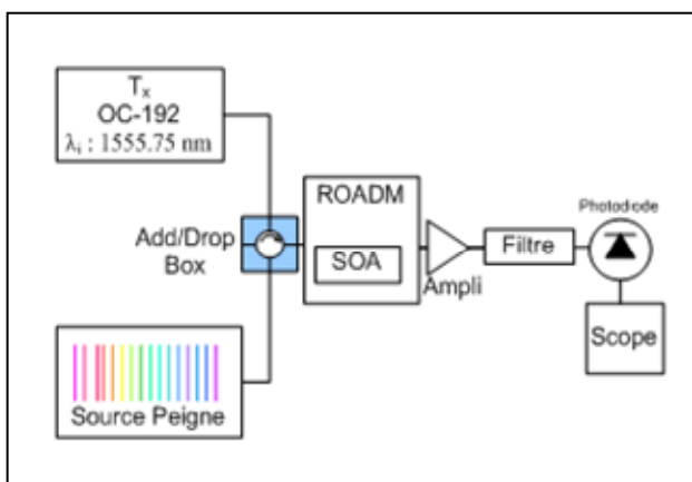
Figure 4.24 Montage 6 : T_x + SP + ROADM + Ampli + Filtre + Pd + BERT 32 \lambda , toutes à travers WB_2 .
