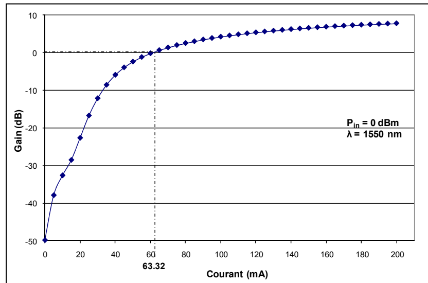
Figure 2.5 Courbe du gain saturé en fonction du courant, P_{in} = 0 dBm.
