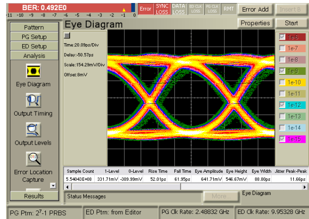
Figure 4.17 Diagramme de l'œil du montage 2.
