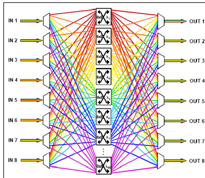
Figure 1.24 Schéma d'un ROADM basé sur un WXC. Tiré d'Eldada (2007)
