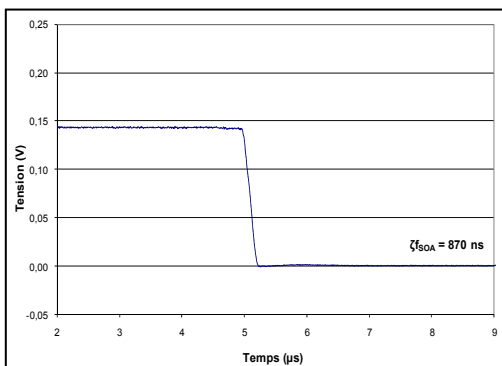
Figure 2.34 Tracé descente à 1μs (cas B).
