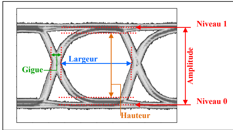
Figure 4.13 Un diagramme de l'œil.
