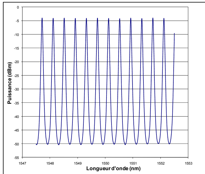
Figure 4.3 Spectre de la source peigne centré autour de 1550 nm, avec une résolution de 0,1 nm.
