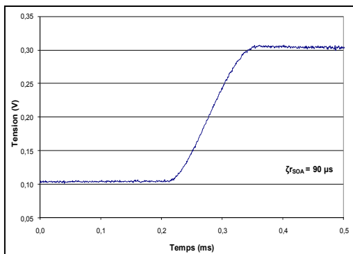
Figure 2.15 Tracé montée à 100µs (cas A).
