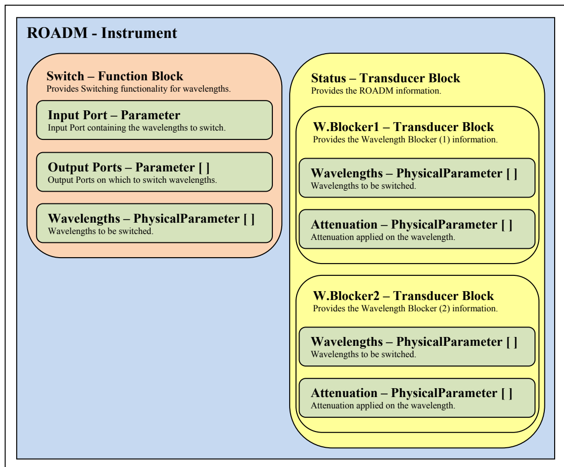
Figure 3.10 Modélisation du ROADM avec GRIM.
