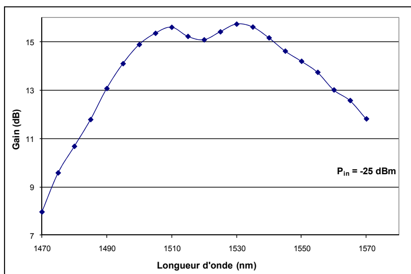
Figure 2.7 Spectre de gain en fonction de la longueur d'onde, à P_{in} = -25 \text{ dBm} .
