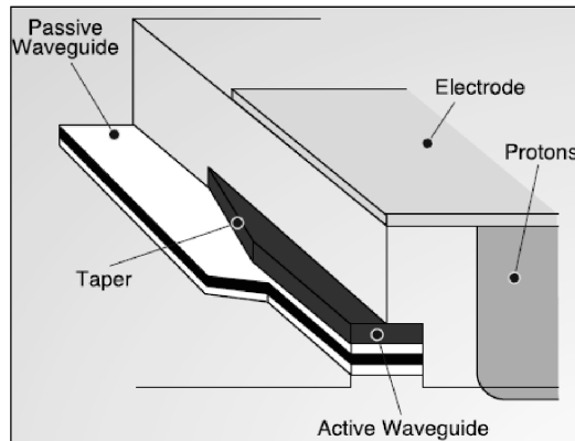
Figure 2.2 Structure de base d'un SOA standard.
