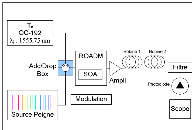
Figure 4.28 Montage 8 : T_x + SP + ROADM + Ampli + Bobine1 + Bobine2 + Filtre + Pd + BERT 31 \lambda à travers WB 1 , 1 \lambda à travers WB 2 .
