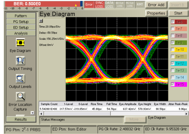
Figure 4.15 Diagramme de l'œil du montage 1.
