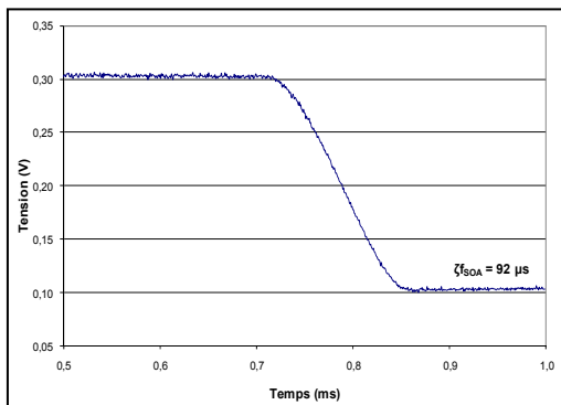
Figure 2.27 Tracé descente à 100µs (cas A).
