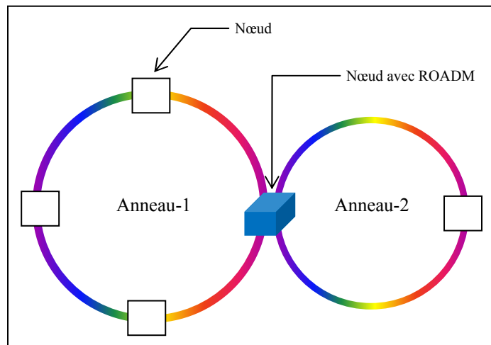
Figure 1.20 Deux réseaux en anneau reliés par un ROADM.
