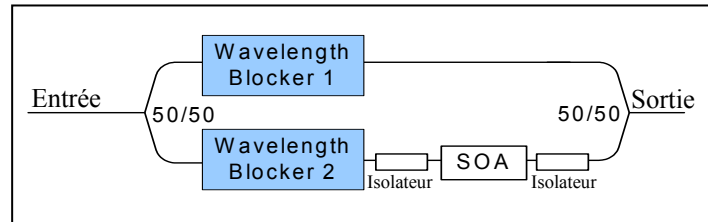
Figure 2.1 ROADM à temps de commutation ajustable.
