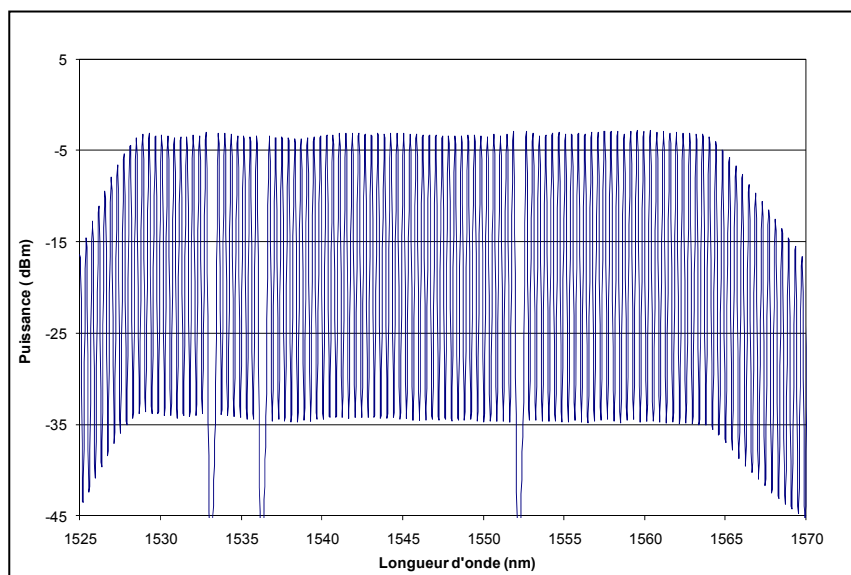
Figure 4.12 Signal à la sortie du module d'insertion/extraction avec le transmetteur à 1555,75 nm activé.
