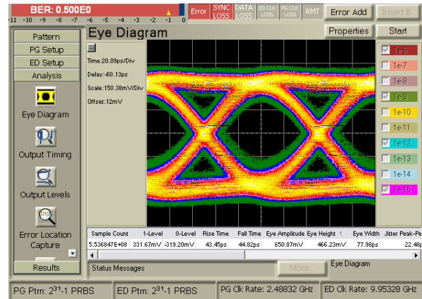
Figure 4.27 Diagramme de l'œil du montage 7.
