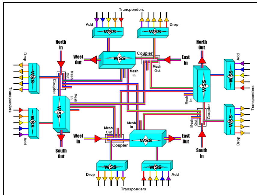
Figure 1.23 Schéma d'un "colorless-WSS-ROADM" de degré 4. Tiré d'Eldada (2007)
