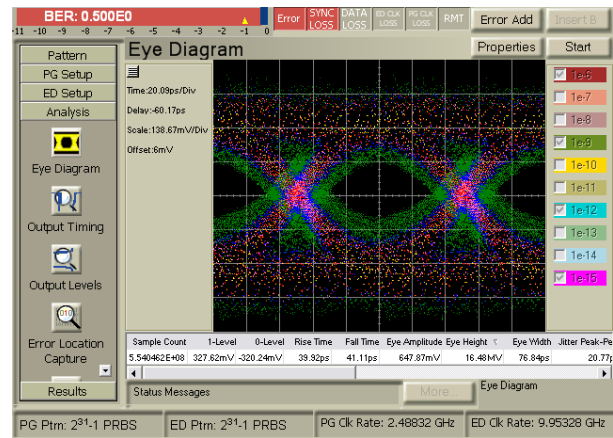
Figure 4.29 Diagramme de l'œil du montage 8.
