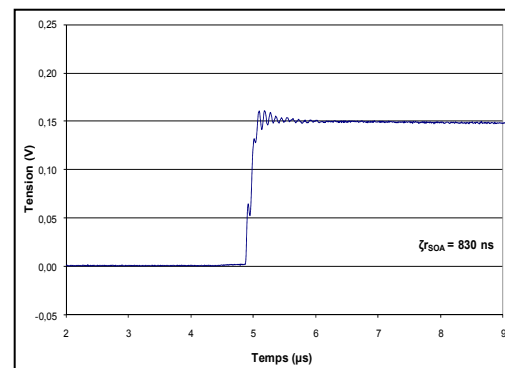
Figure 2.23 Tracé montée à 1µs (cas C).
