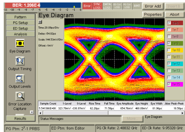
Figure 4.19 Diagramme de l'œil du montage 3.
