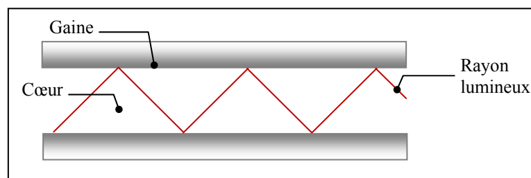
Figure 1.7 Réflexion totale interne due à la différence d'indices de réfraction. Tiré de Camisard (2007)
