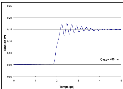
Figure 2.25 Tracé montée à 100ns (cas B).
