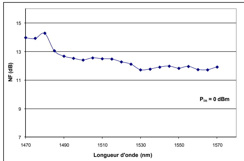
Figure 2.12 Spectre de figure de mérite en fonction de la longueur d'onde, à P_{in} = 0 dBm.
