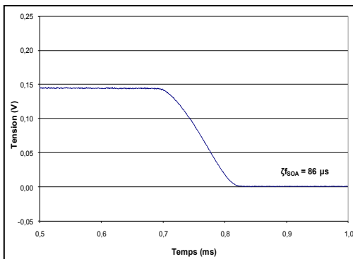
Figure 2.28 Tracé descente à 100µs (cas B).
