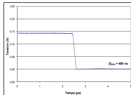
Figure 2.38 Tracé descente à 100ns (cas C).
