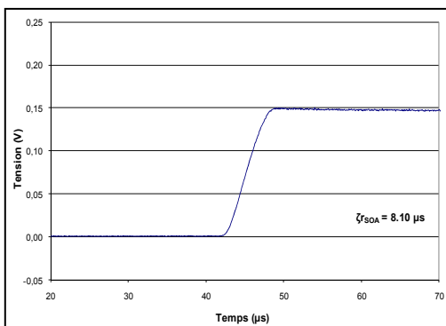
Figure 2.19 Tracé montée à 10µs (cas B).
