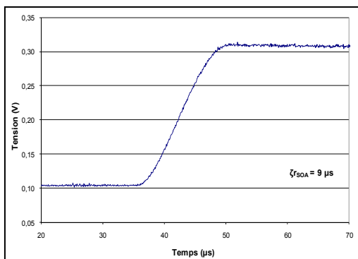
Figure 2.18 Tracé montée à 10µs (cas A).
