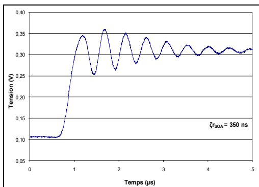
Figure 2.24 Tracé montée à 100ns (cas A).
