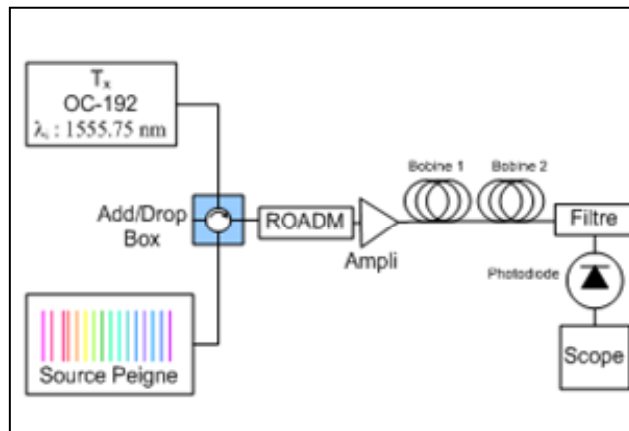
Figure 4.22 Montage 5 : T_x + SP + ROADM + Ampli + Bobine1 + Bobine2 + Filtre + Pd + BERT 32 \lambda , toutes à travers WB_1 .
