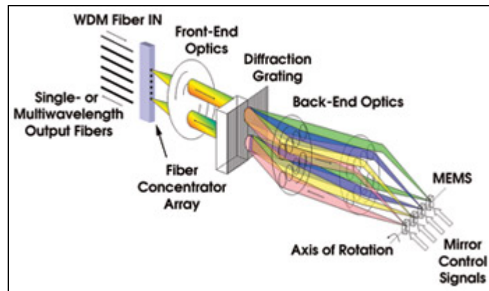
Figure 1.17 "Wavelength Selective Switch" à base de MEMS. Tiré de Nagy (2006)
