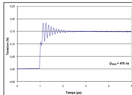
Figure 2.26 Tracé montée à 100ns (cas C).
