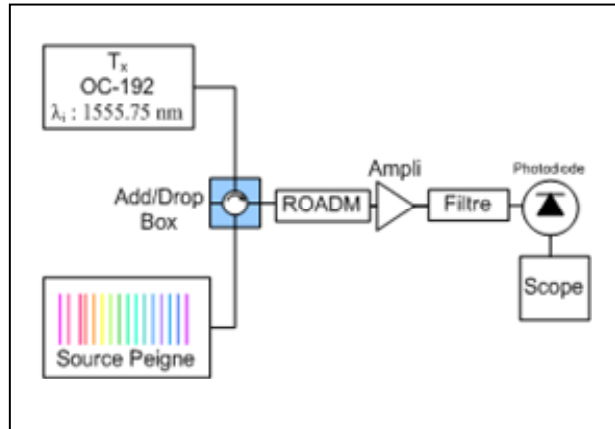
Figure 4.20 Montage 4 : T_x + SP + ROADM + Ampli + Filtre + Pd + JBERT 32 \lambda , toutes à travers WB_1 .
