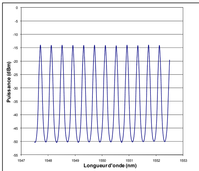
Figure 4.7 Toutes les longueurs d'onde atténuées de 10 dB.
