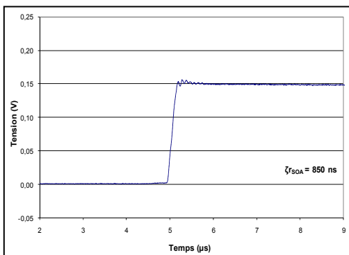
Figure 2.22 Tracé montée à 1µs (cas B).
