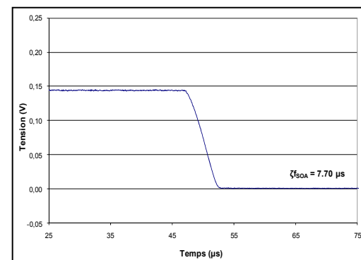
Figure 2.32 Tracé descente à 10µs (cas C).
