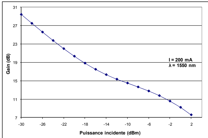
Figure 2.6 Courbe du gain en fonction de la puissance incidente.
