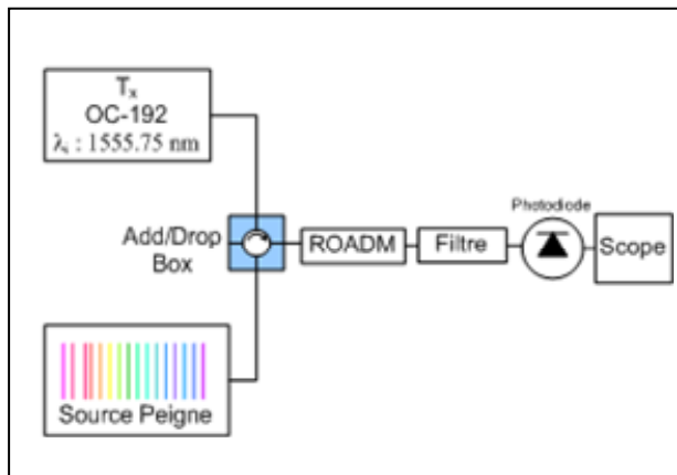
Figure 4.18 Montage 3 : T_x + SP + ROADM + Filtre + Pd + JBERT 32 \lambda , toutes à travers WB_1 .
