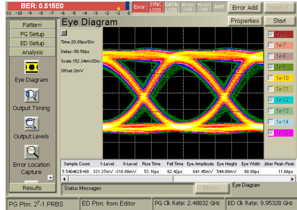
Figure 4.21 Diagramme de l'œil du montage 4.
