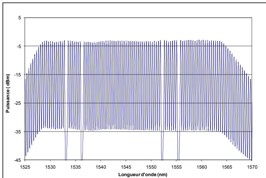
Figure 4.11 Signal à la sortie du module d'insertion/extraction avec le transmetteur à 1555,75 nm désactivé.
