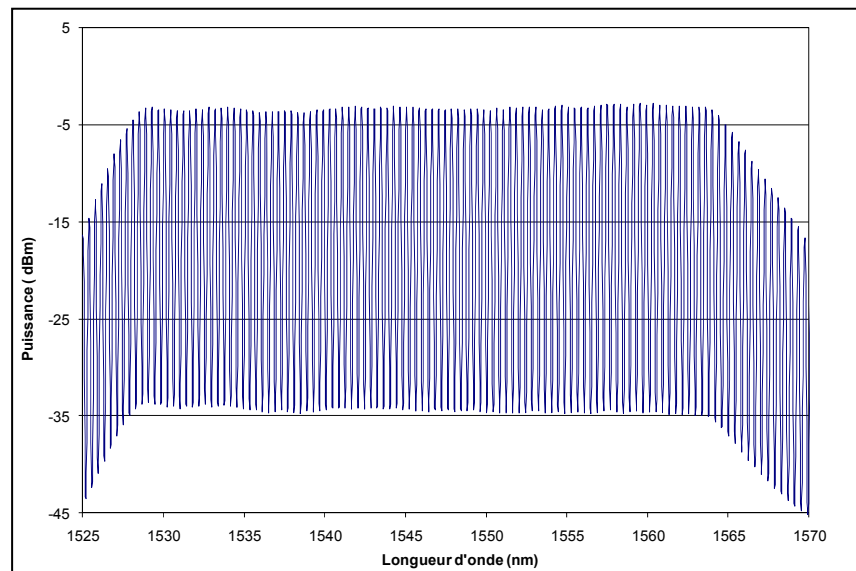
Figure 4.2 Spectre de la source peigne sans atténuations.
