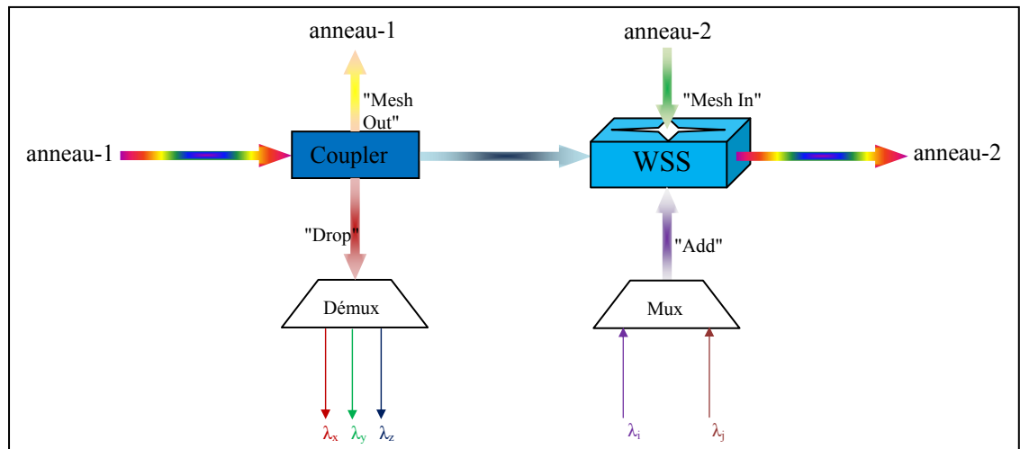
Figure 1.21 Schéma d'un WSS-ROADM coloré. Adapté d'Eldada (2007)
