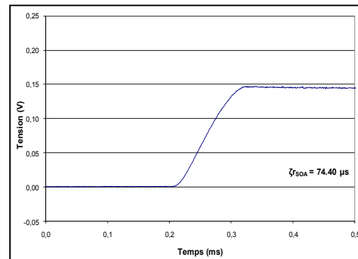
Figure 2.17 Tracé montée à 100µs (cas C).
