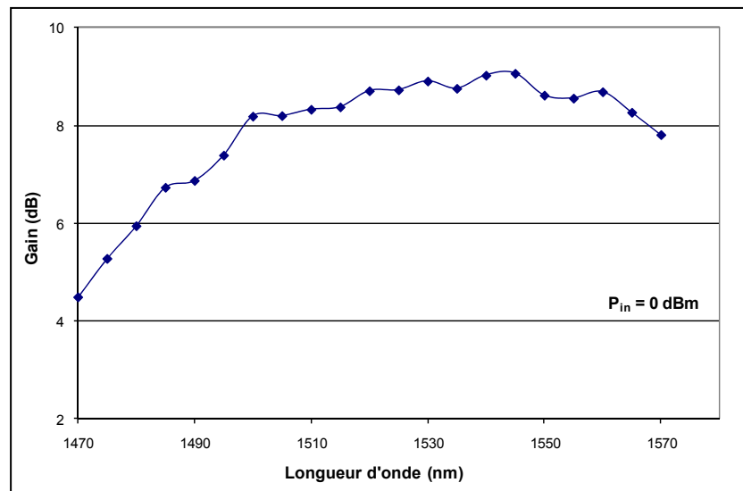
Figure 2.8 Spectre de gain en fonction de la longueur d'onde, à P_{in} = 0 dBm.
