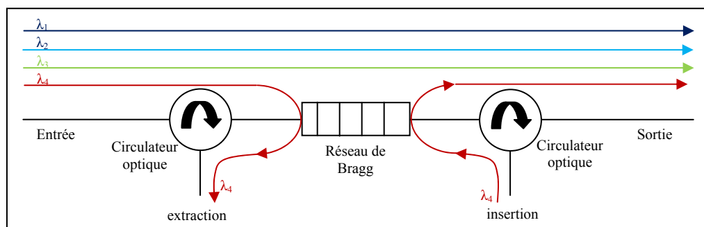
Figure 1.15 Schéma d'un OADM.
