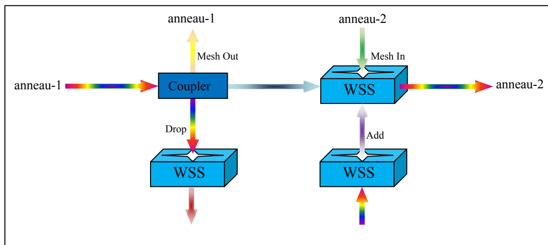
Figure 1.22 Schéma d'un "colorless-WSS-ROADM".
