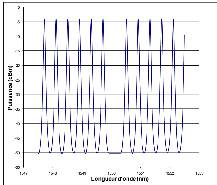
Figure 4.5 La longueur d'onde 1550.12 nm est bloquée.
