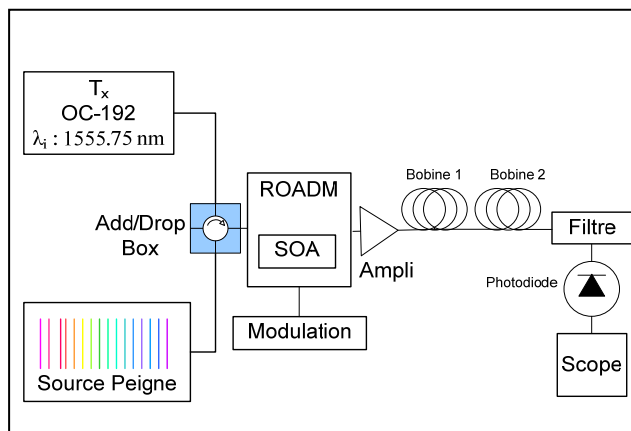
Figure 4.30 Montage 9 : T_x + SP + ROADM + Ampli + Bobine1 + Bobine2 + Filtre + Pd + BERT 3 \lambda à travers WB 1 , 29 \lambda à travers WB 2 .
