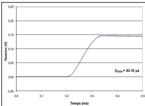
Figure 2.16 Tracé montée à 100µs (cas B).
