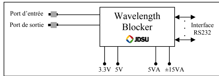
Figure 2.39 Diagramme fonctionnel du WB de JDSU.
