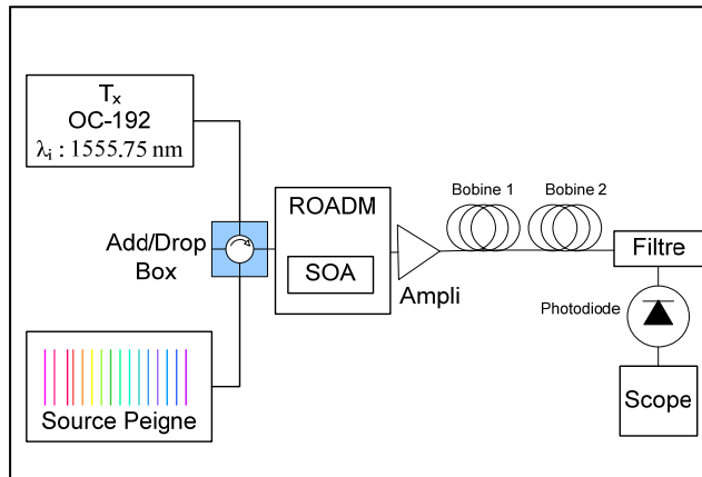
Figure 4.26 Montage 7 : T_x + SP + ROADM + Ampli + Bobine1 + Bobine2 + Filtre + Pd + BERT 32 \lambda , toutes à travers WB 2 , Ampli en AGC.
