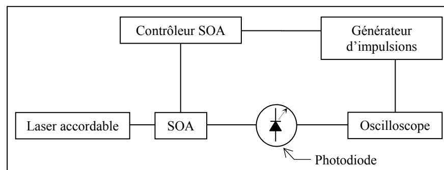
Figure 2.14 Montage expérimental de caractérisation du SOA en modulation.
