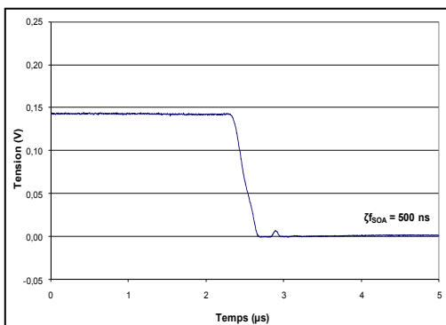
Figure 2.37 Tracé descente à 100ns (cas B).
