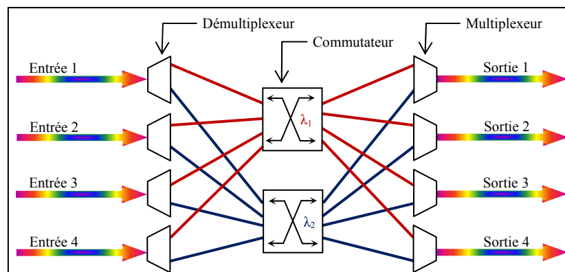
Figure 1.18 "Wavelength Cross Connect" de 4 fibres de 2 canaux. Adapté d'Eldada (2007)
