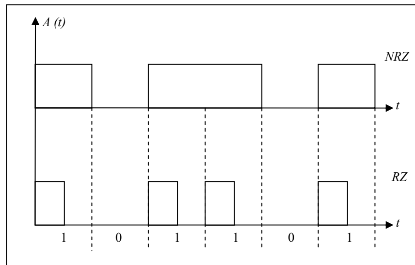
Figure 1.5 Modulation NRZ et RZ.
