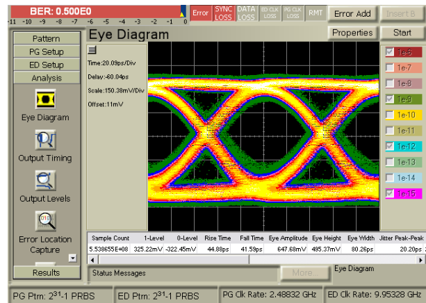
Figure 4.23 Diagramme de l'œil du montage 5.
