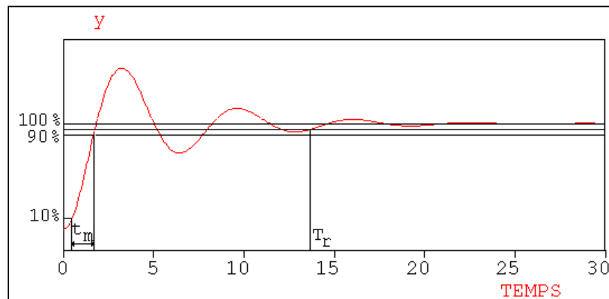
Figure 2.13 Temps de montée.
