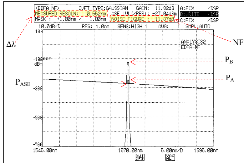
Figure 2.10 Calcul du NF sur l'OSA pour \lambda = 1570 nm.
