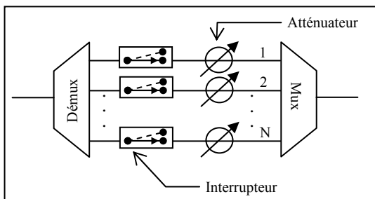
Figure 1.16 Un Wavelength Blocker. Adapté d'Eldada (2007)
