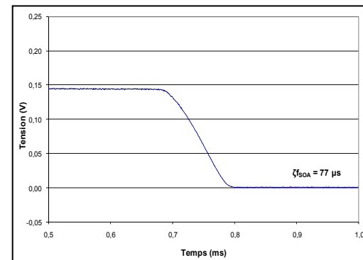
Figure 2.29 Tracé descente à 100µs (cas C).
