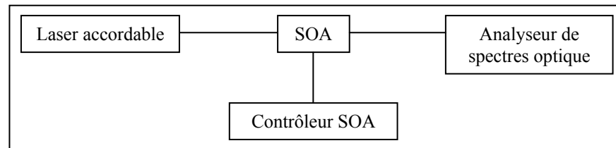
Figure 2.9 Montage expérimental de caractérisation du SOA (figure de mérite).
