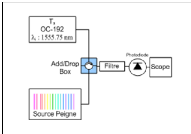
Figure 4.16 Montage 2 : T_x + SP + Filtre + Pd + JBERT.
