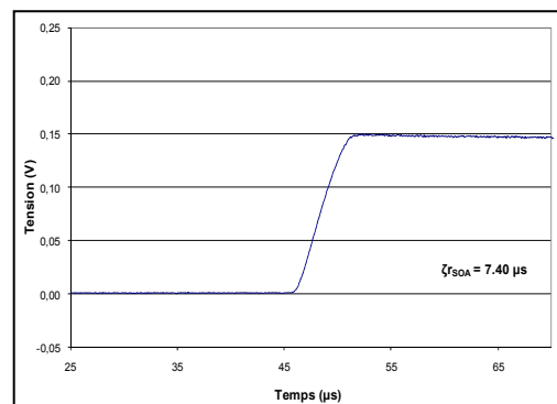
Figure 2.20 Tracé montée à 10µs (cas C).
