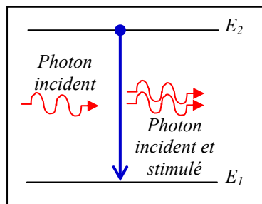
Figure 1.10 L'émission stimulée.
