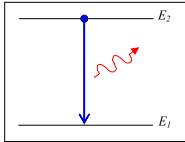
Figure 1.12 L'émission spontanée. Tiré de Kasap (2001)
