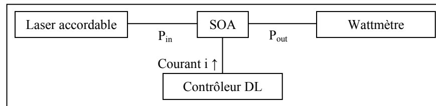
Figure 2.3 Montage expérimental de caractérisation du SOA (gain).
