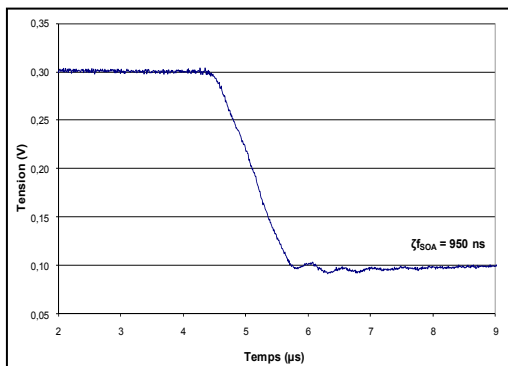
Figure 2.33 Tracé descente à 1μs (cas A).
