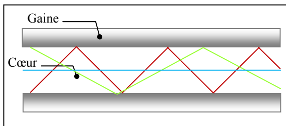
Figure 1.8 Propagation de la lumière dans une fibre multimode.
