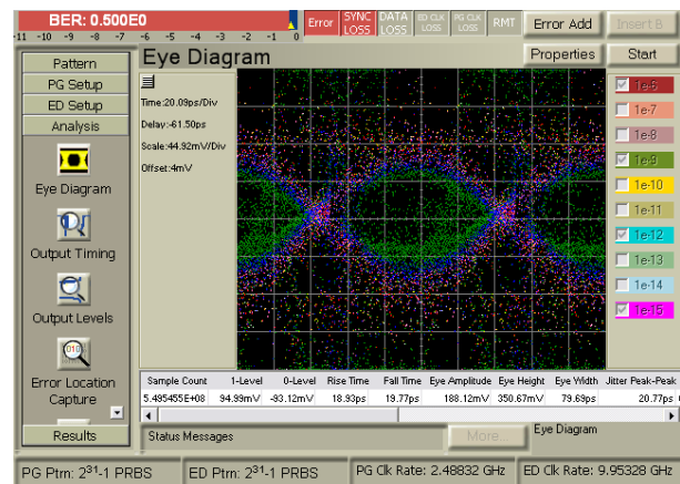
Figure 4.31 Diagramme de l'œil du montage 9.
