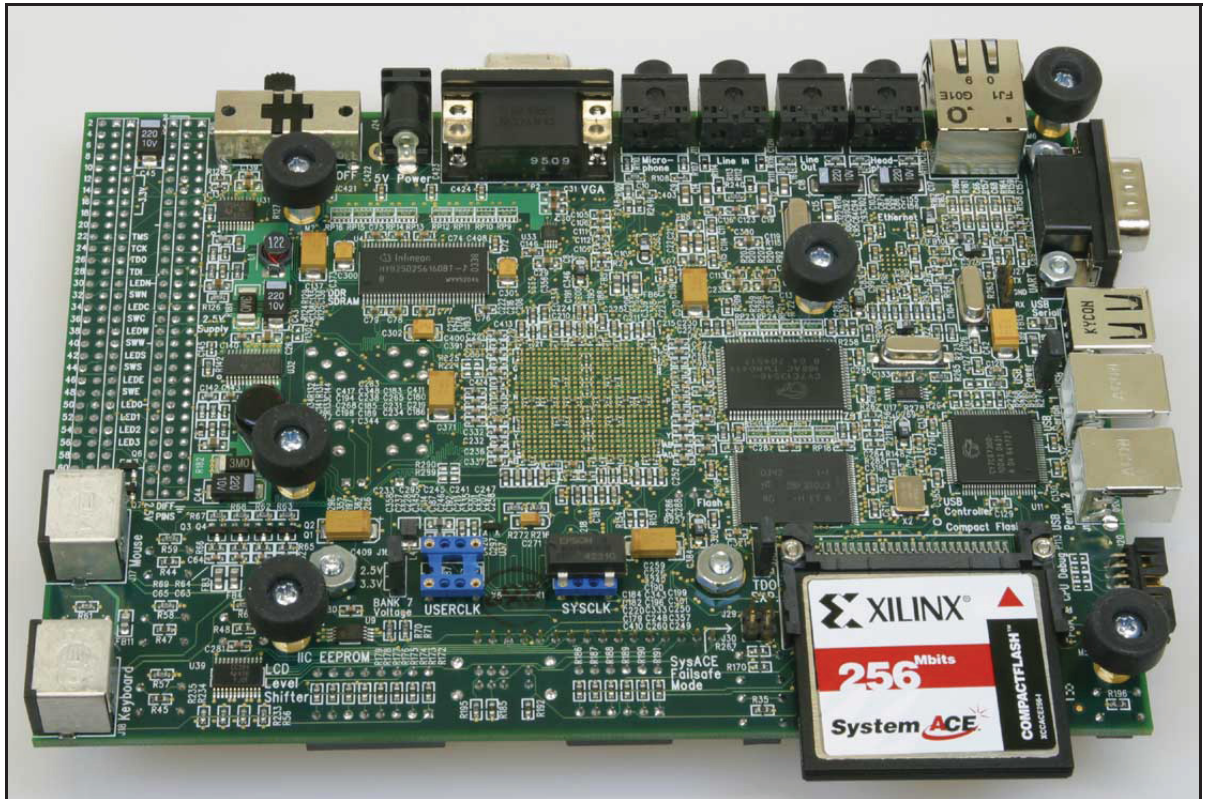
Figure 2.4 Carte Xilinx ML403 (verso).
