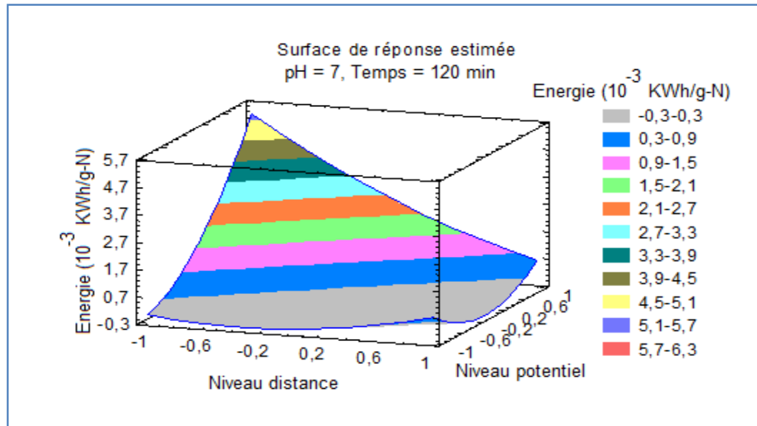
Figure 3.16 Effet de l'interaction distance-potential sur la consommation d'énergie (électrodes en acier inoxydable).
