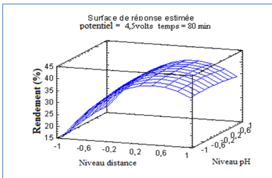
A.III.1 Le rendement en fonction du pH et la distance.
