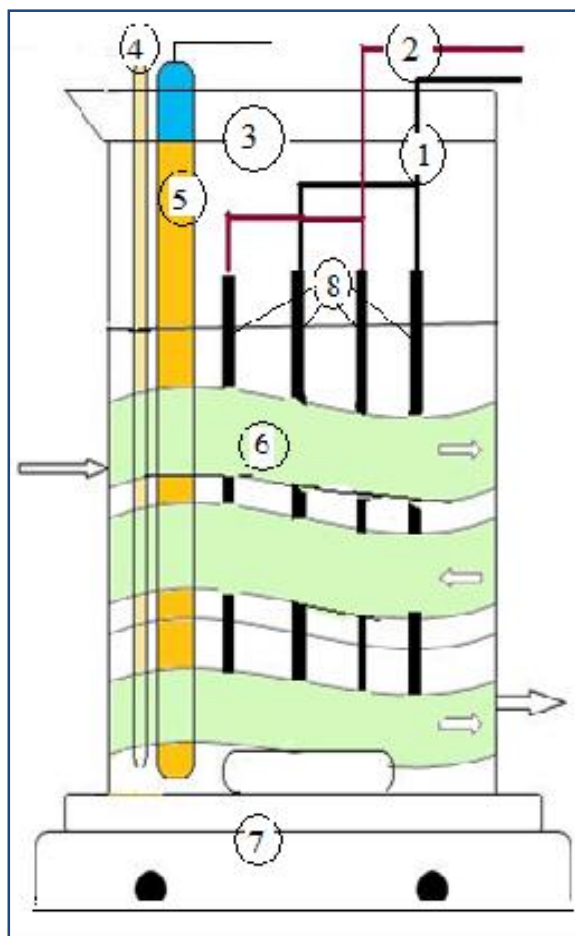
Figure 2.1 Dispositif expérimental.
