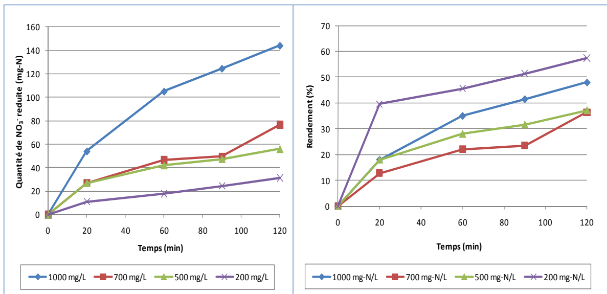
Figure 3.9 Rendement sur acier inoxydable en fonction de la concentration initiale (d = 5 mm; potentiel = 4,0 V; v = 300 mL).
