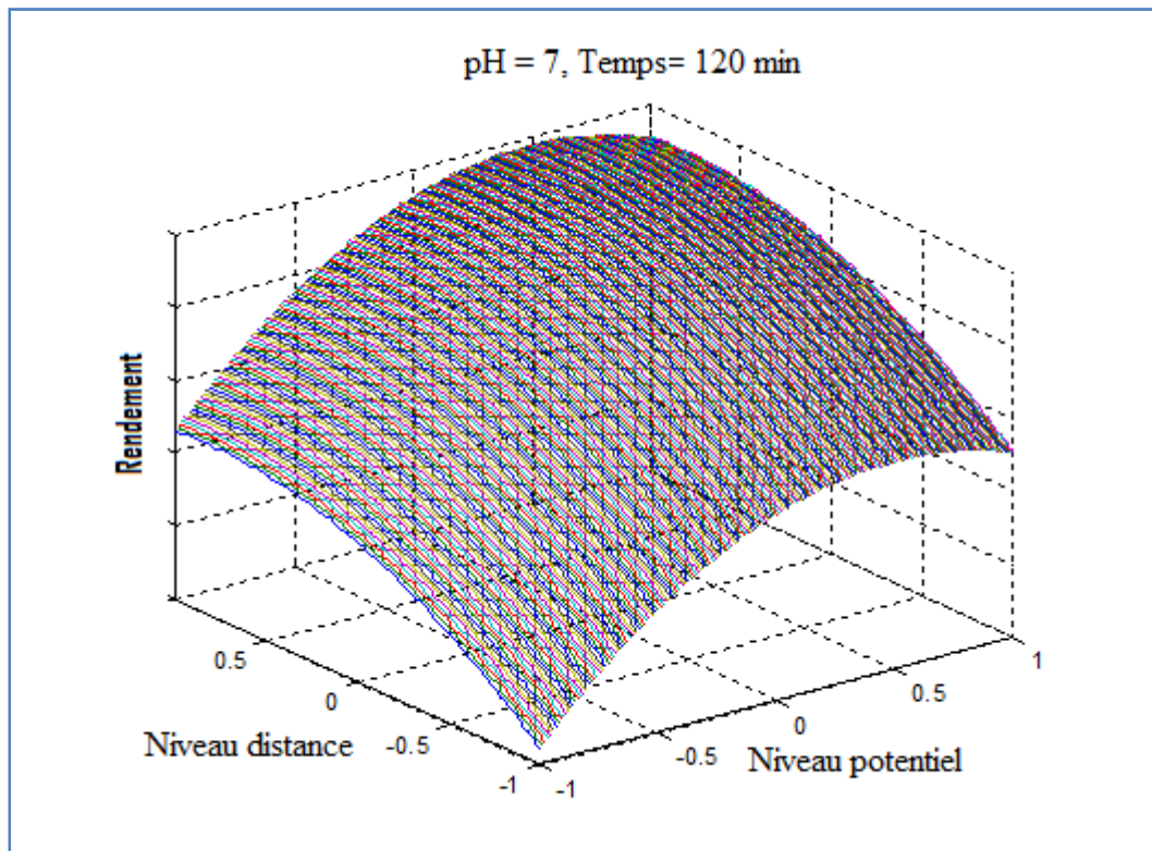
Figure 3.17 Variation du rendement pour un pH de 7 et un temps de 120 min (électrodes en acier inoxydables).
