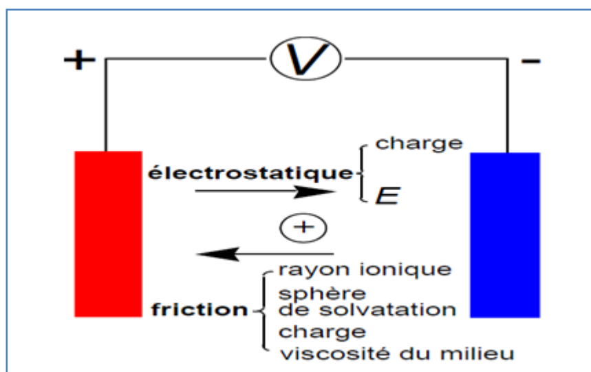
Figure 1.5 Forces qui influent le déplacement des ions. Adapté de Atkins et De Paula (2004)
