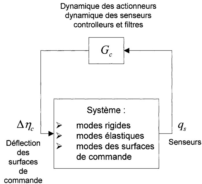
Figure 8 Le système aéroservoélastique en boucle fermée
