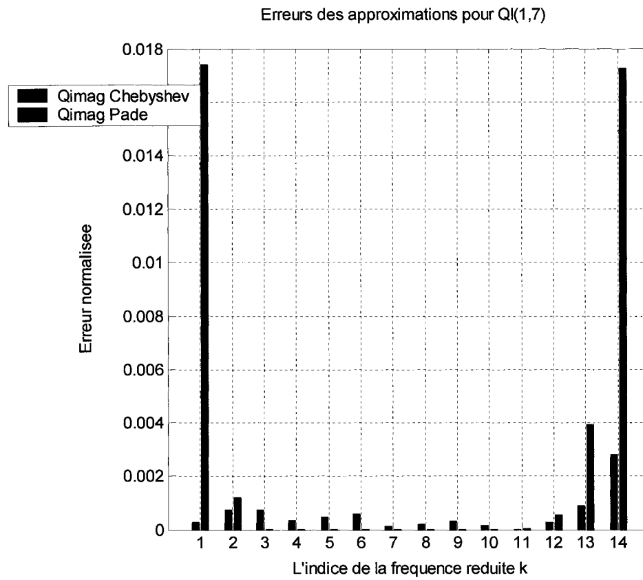
Graphique 7 Erreurs normalisées d'approximation pour Q_I(1,7) versus les fréquences réduites k
