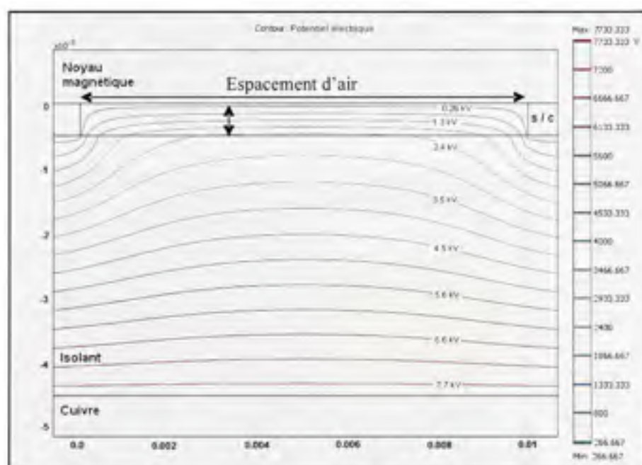
Figure 2.4 Les surfaces équipotentiellles développées dans l'isolant ainsi que dans l'espace d'air.
