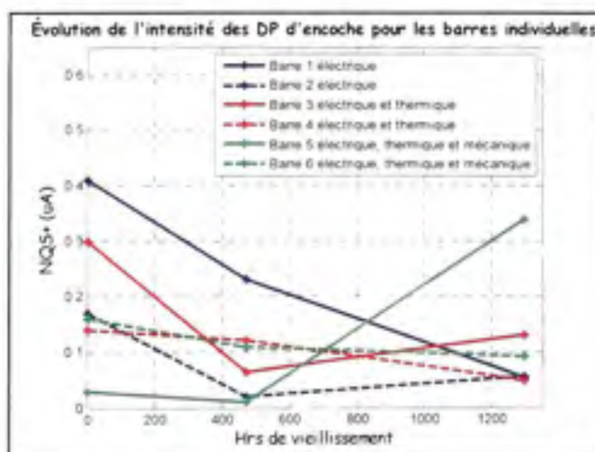
Figure 5.14 L'évolution du paramètre NQS+ pour les barres individuelles.
