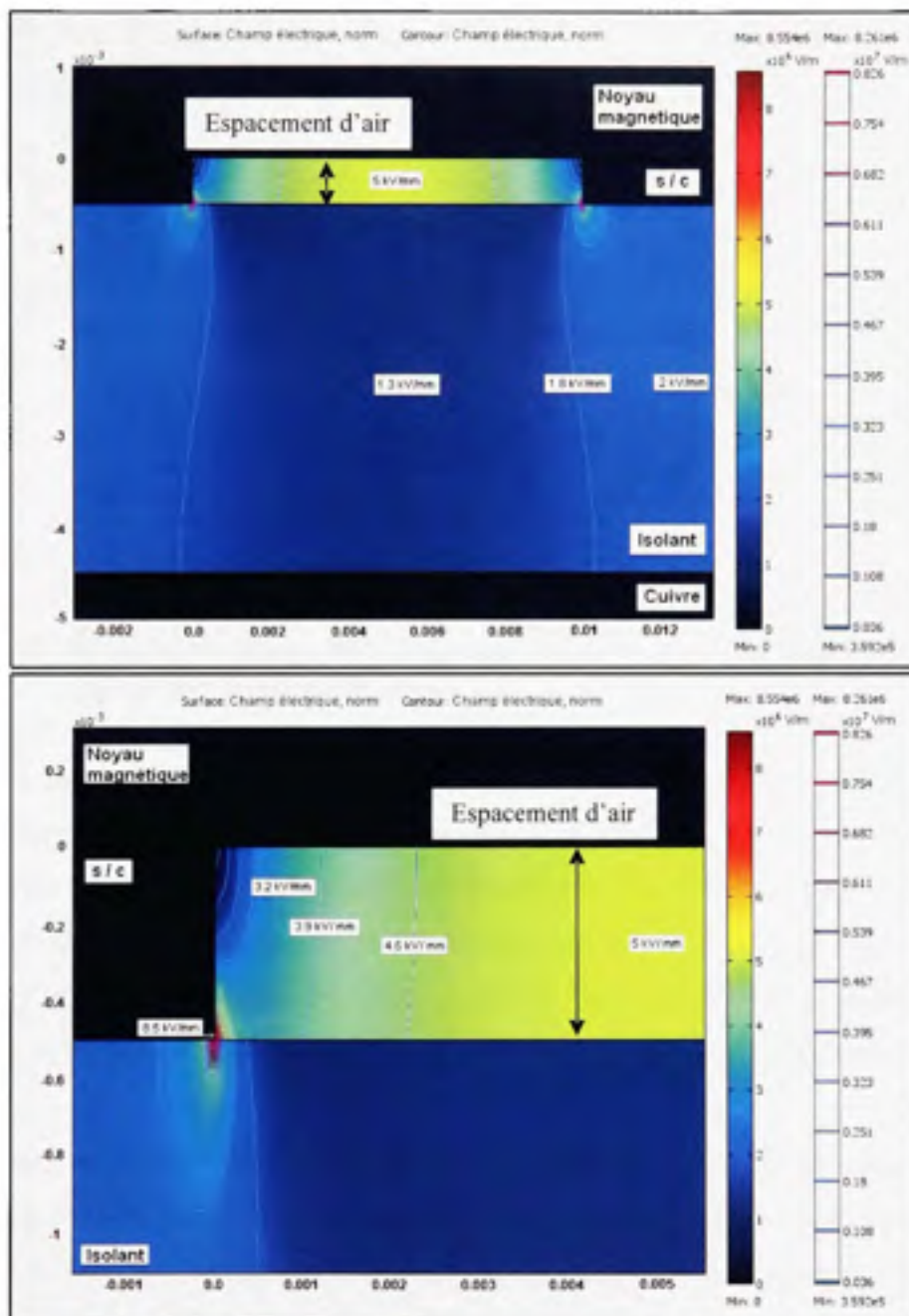
Figure 2.5 La grandeur du champ électrique dans l'isolant et dans l'espaceur d'air (en haut) et un agrandissement dans l'espaceur d'air (en bas).
