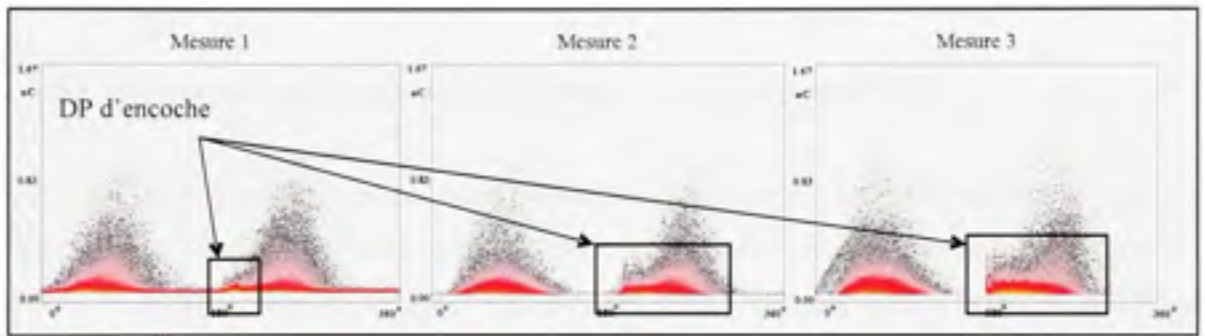
Figure 4.6 Les patrons PRPD des barres en groupe à l'ambient avec gain de 10-40.
