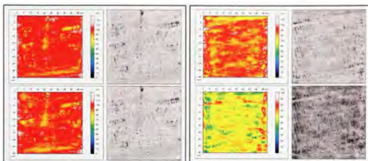
Figure 4.29 Les profils de surface de la mesure 1 (haut) et la mesure 3 (bas) pour la barre 1 (gauche) et de la barre 2 (droite).
