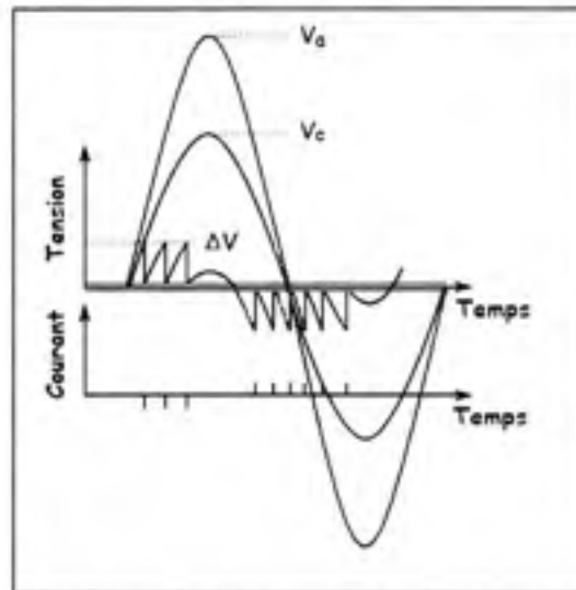
Figure 4.2 L'activité de DP durant un cycle de la tension d'alimentation.
