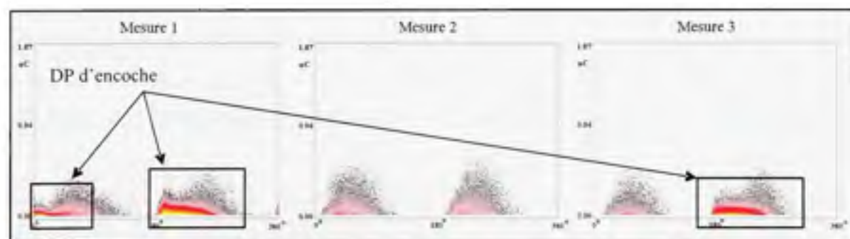
Figure 4.10 Les patrons PRPD mesurés sur la barre 3 en fonction du vieillissement.
