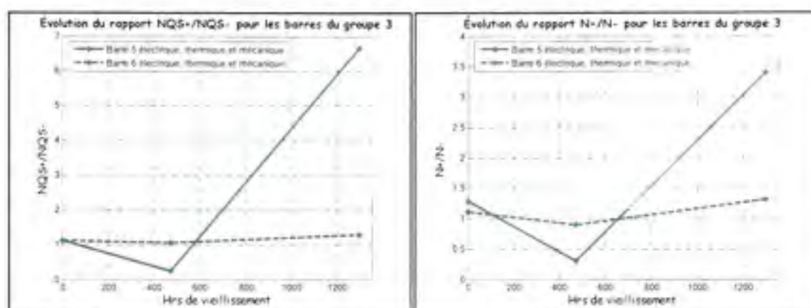
Figure 5.10 L'évolution des ratios NQS et N en fonction du vieillissement pour les barres du groupe 3.
