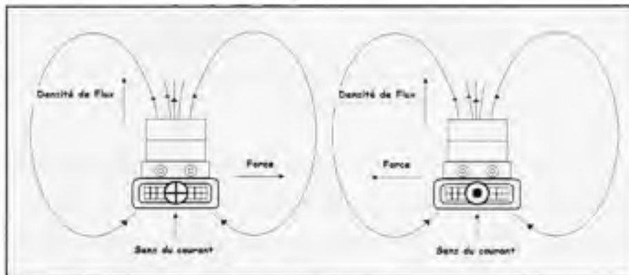
Figure 3.12 Le sens de la force donné par l'interaction du courant induit avec les aimants permanents.
