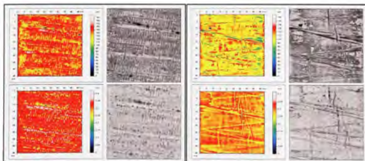
Figure 4.30 Les profils de surface de la mesure 1 (haut) et la mesure 3 (bas) pour la barre 3 (gauche) et de la barre 4 (droite).
