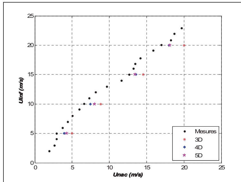
Figure I.1 Résultats des différentes simulations obtenues pour une éolienne opérant dans le sillage placée à 3,4 et 5D, K=25 , modèle k - \epsilon standard.
