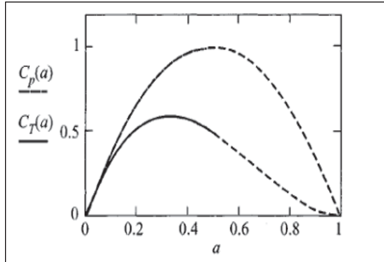
Figure 2.5 Variation de C_P et C_T en fonction du Facteur d'induction a .
