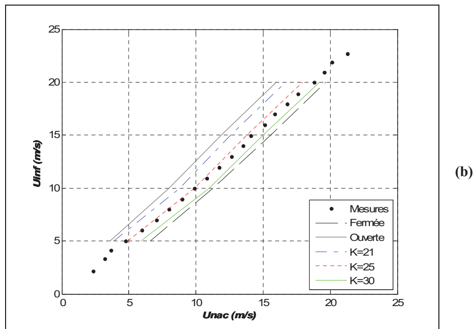
Figure 6.7 Comparaison entre les résultats des simulations et les données expérimentales pour différentes valeurs de K : éolienne isolée, modèle k - \epsilon standard (a) rotor à l'arrêt (b) rotor en marche.
