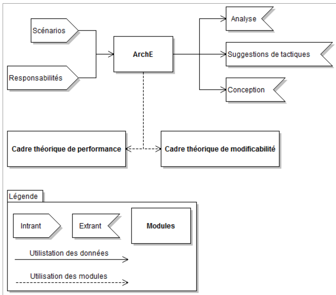
Figure 1.3 Résumé des composantes d'ArchE.
