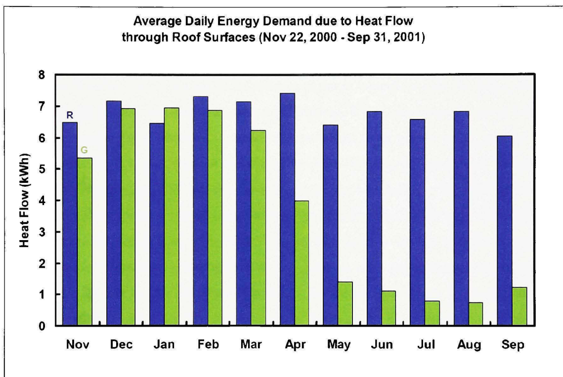
Figure 2.5 FRF - Demande énergétique.
