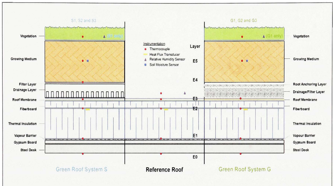
Figure 2.11 ENCC - Coupe typique des systèmes de toit vert étudiés.
