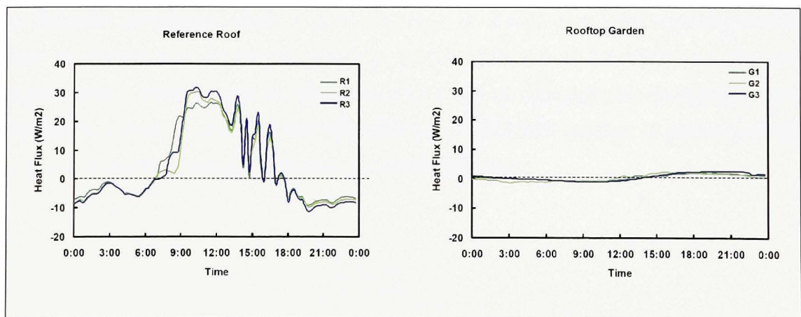
Figure 2.4 FRF – Flux de chaleur pénétrant le toit (16 juillet 2001).
