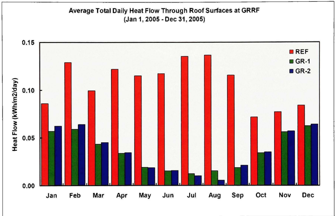
Figure 2.10 GRRF – Demande énergétique pour l'année 2005. Tirée de Connelly et Liu (2006, p. 53)
