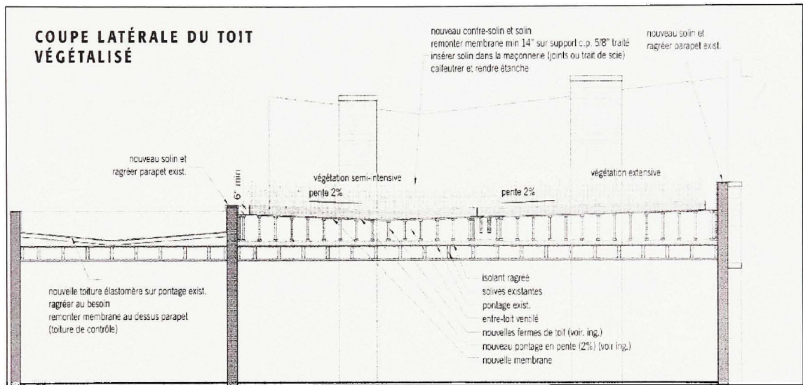
Figure 3.1 Structure du toit du CEU de Montréal.
