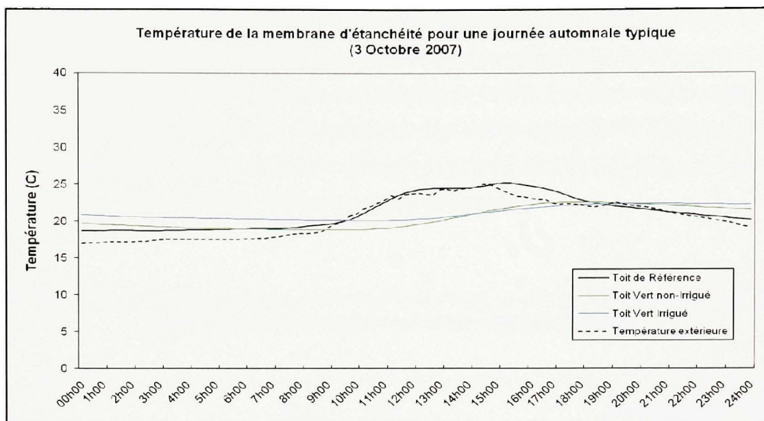
Figure 4.1 Température enregistrée au niveau de la membrane d'étanchéité pour une journée automnale typique.
