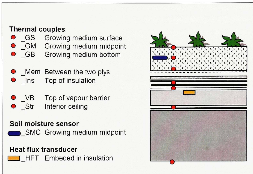
Figure 2.6 GRRF – coupe typique et position des sondes.
