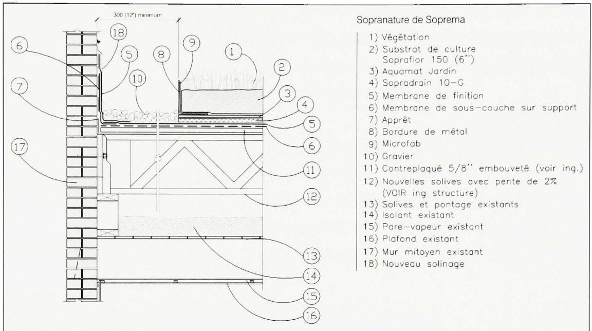
Figure 3.3 Coupe typique du toit du CEU de Montréal.
