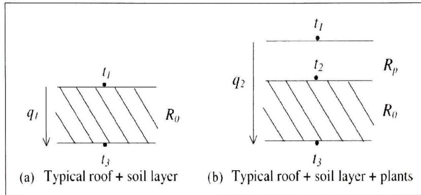
Figure 2.17 Valeur R de la couche de plantes.
