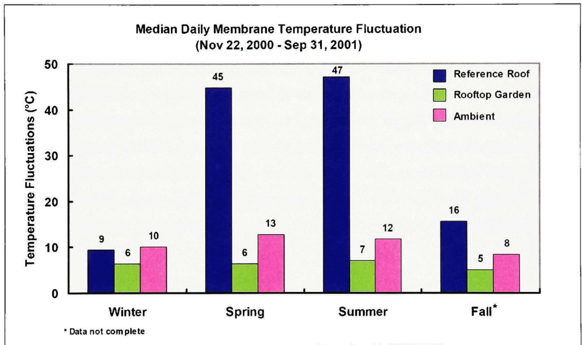
Figure 2.3 FRF – Fluctuation de la température au niveau de la membrane d'étanchéité.
