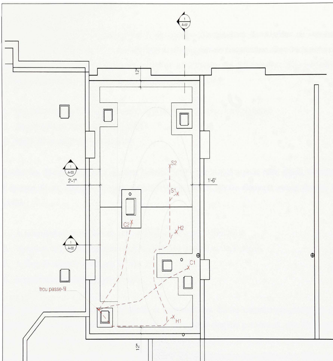
Figure 3.8 Position des sondes du toit du CEU de Montréal.
