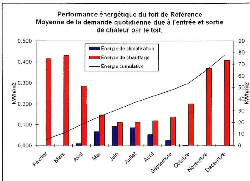
Figure 4.12 Toit de Référence - demande d'énergie due à l'entrée et sortie de chaleur par le toit.
