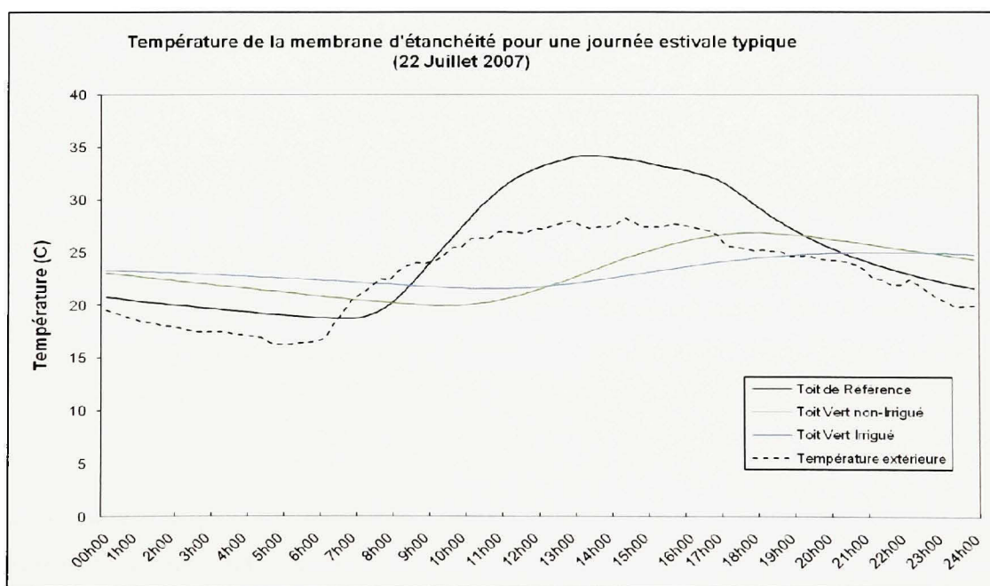
Figure 4.2 Température enregistrée au niveau de la membrane d'étanchéité pour une journée estivale typique.
