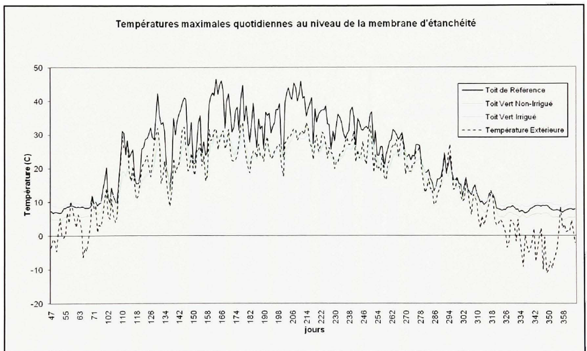
Figure 4.3 Températures maximales quotidiennes au niveau de la membrane d'étanchéité.
