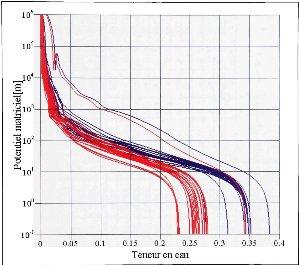
Figure 4.1 Courbes de rétention (Arya-Paris en bleu) et courbes corrigées (en rouge).
