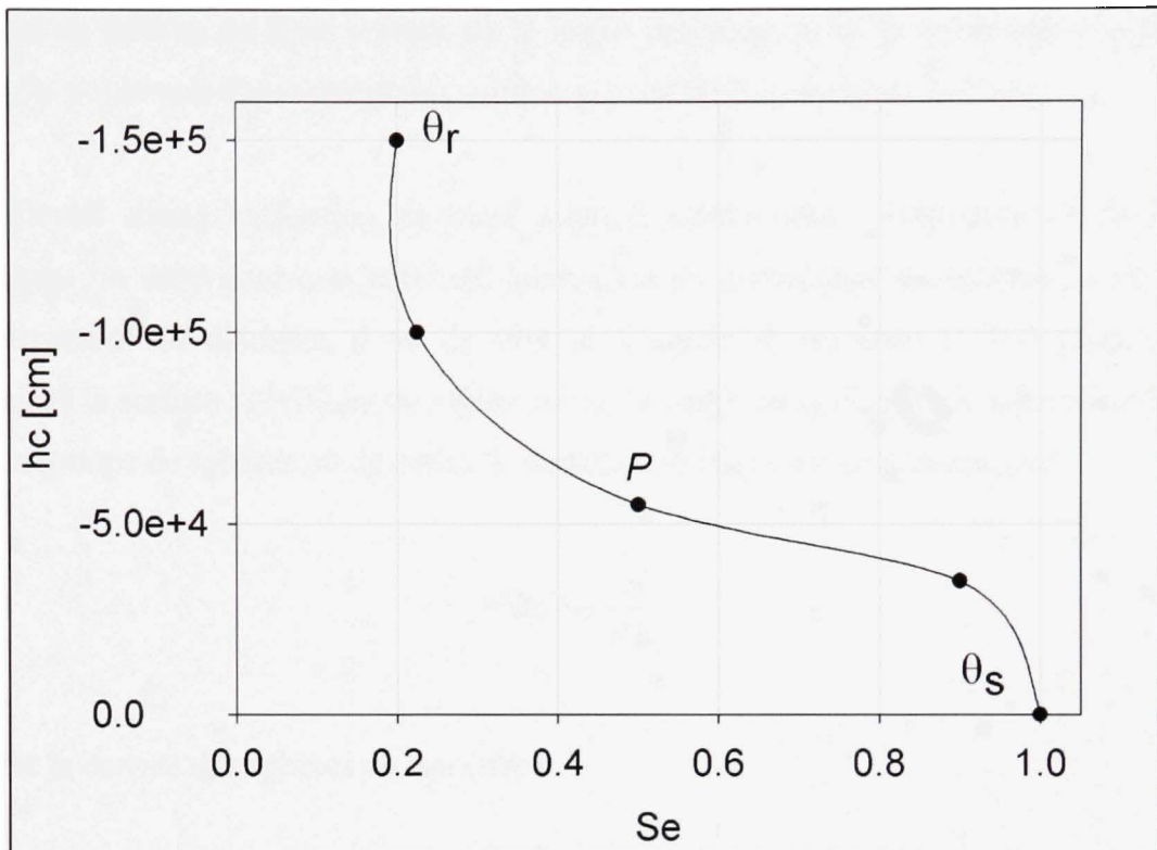
Figure 2.4 Détermination graphique des paramètres de van Genuchten.
