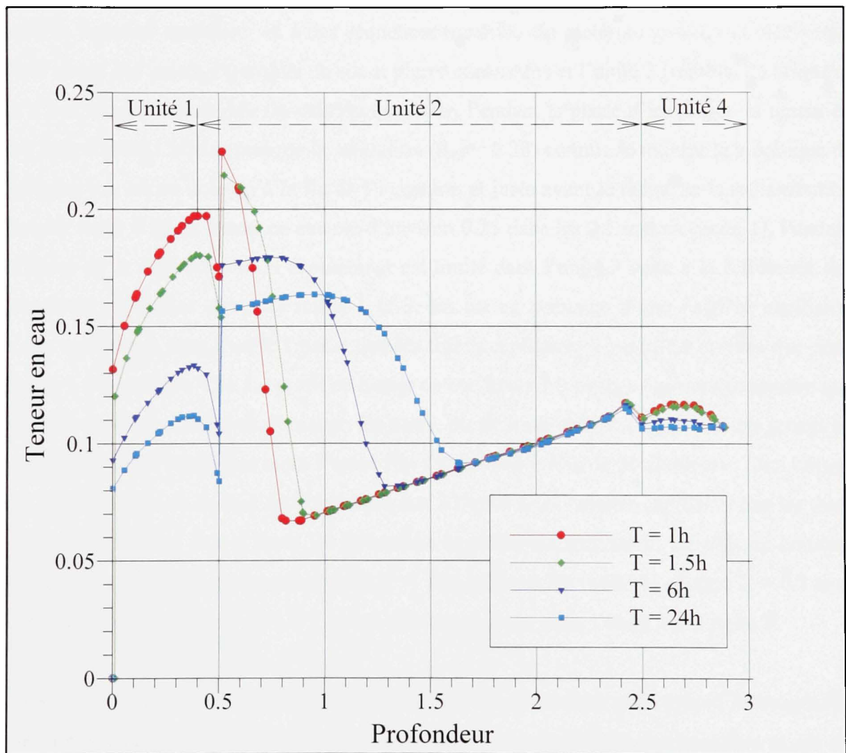
Figure 4.9 Profil de teneurs en eau à X = 1.5\text{m} .
