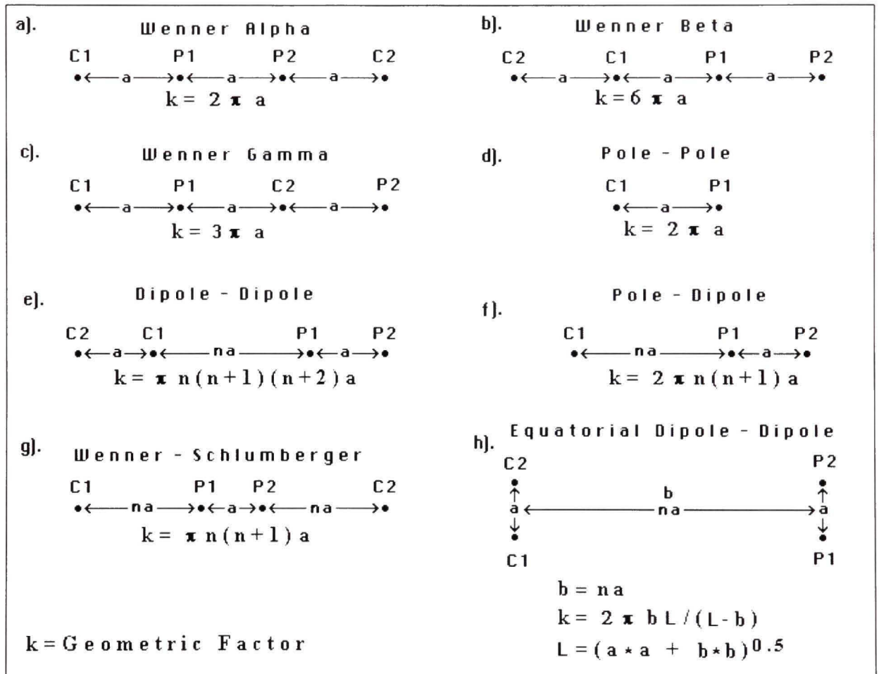
Figure 1.5 Configuration des électrodes.
