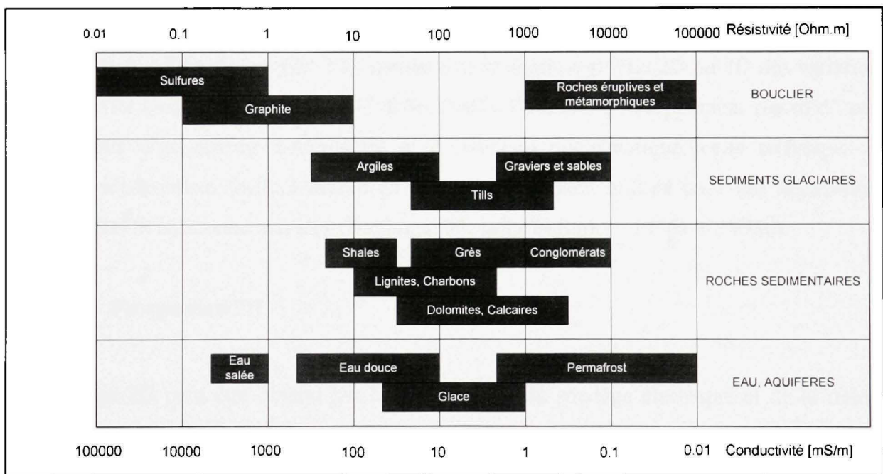
Figure 1.4 Résistivités et conductivités des sédiments, roches et eaux.
