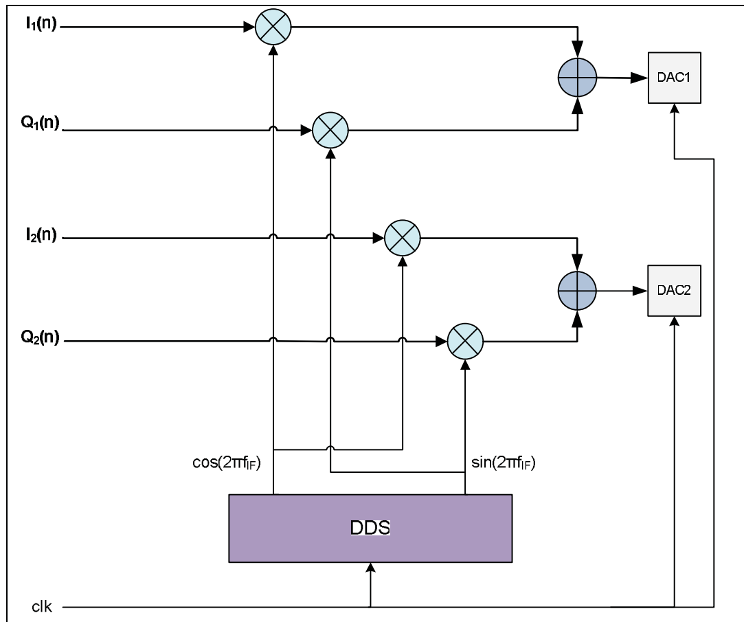
Figure 2.28 Architecture du bloc modulateur I/Q numérique.
