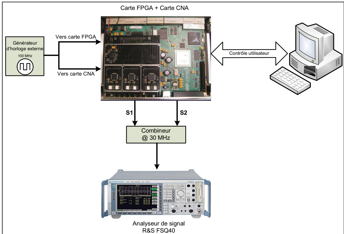
Figure 2.35 Plateforme des tests numériques.
