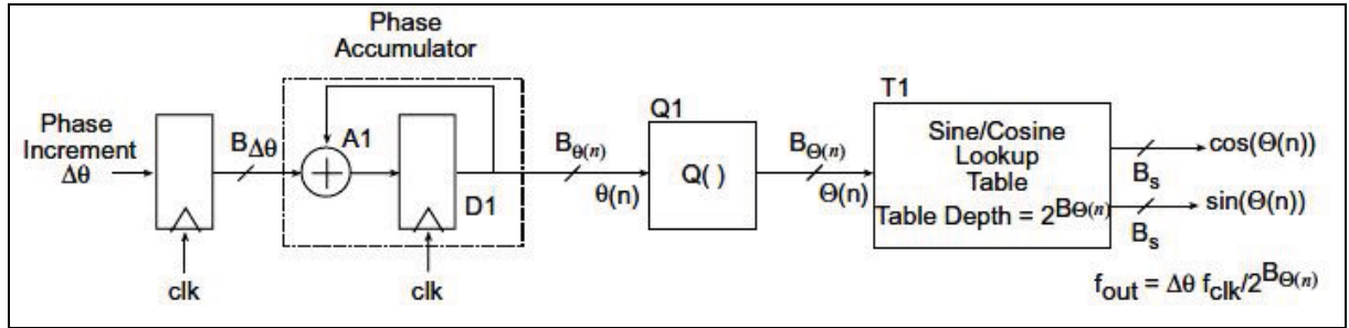
Figure 2.29 Shéma bloc du DDS.
