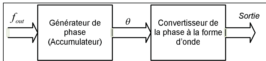
Figure 2.14 Processus fondamental d'un DDS.
