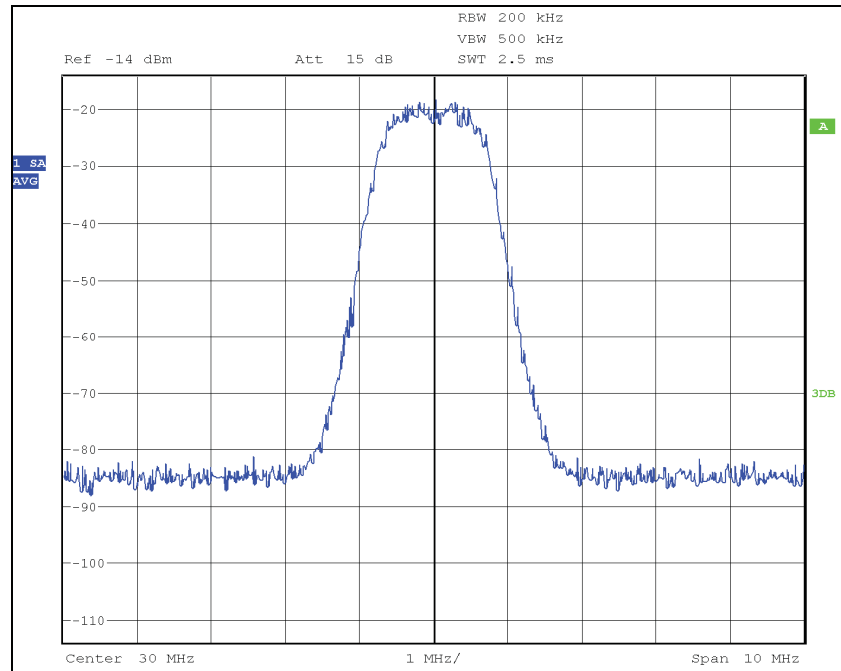
Figure 2.37 Spectre du signal S pour un taux de symboles de 1.25 MHz.
