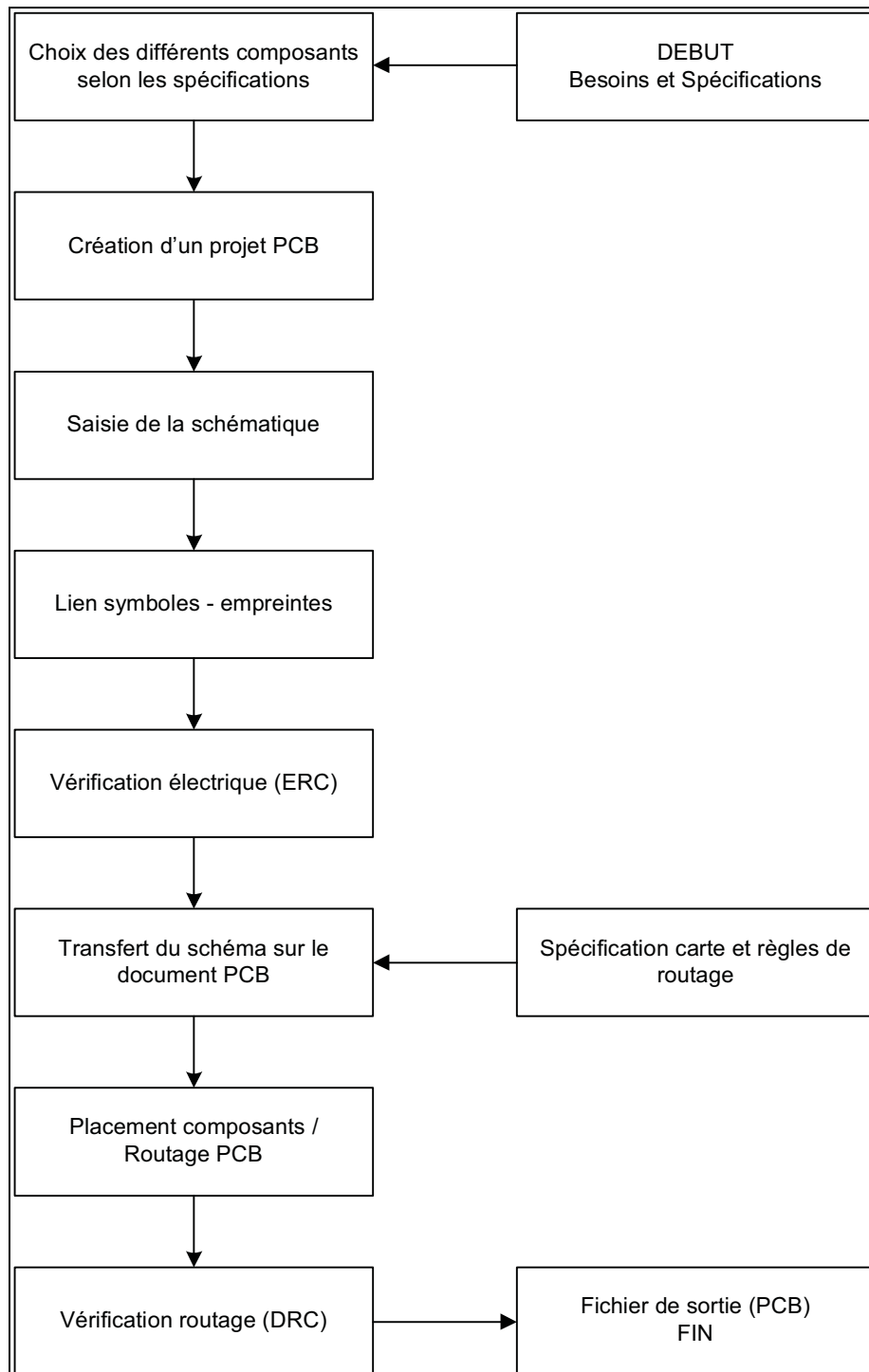
Figure 3.5 Flot de conception de la carte électronique.
