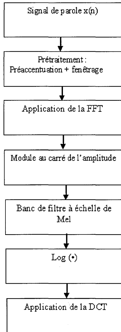
Figure 19 Processus pour l'obtention des coefficients MFCCs
