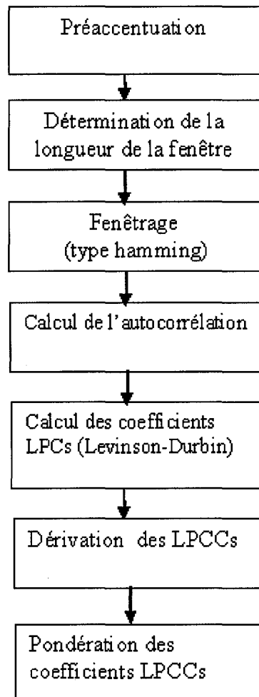
Figure 27 Processus de l'extraction des paramètres LPCCs pondérés
