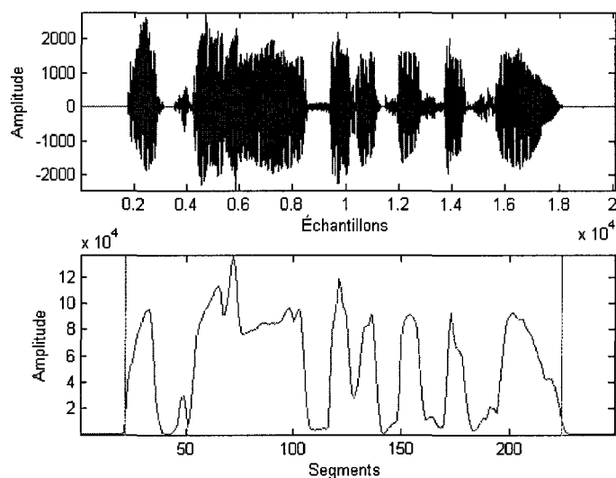
Figure 46 Détection des points début et fin
