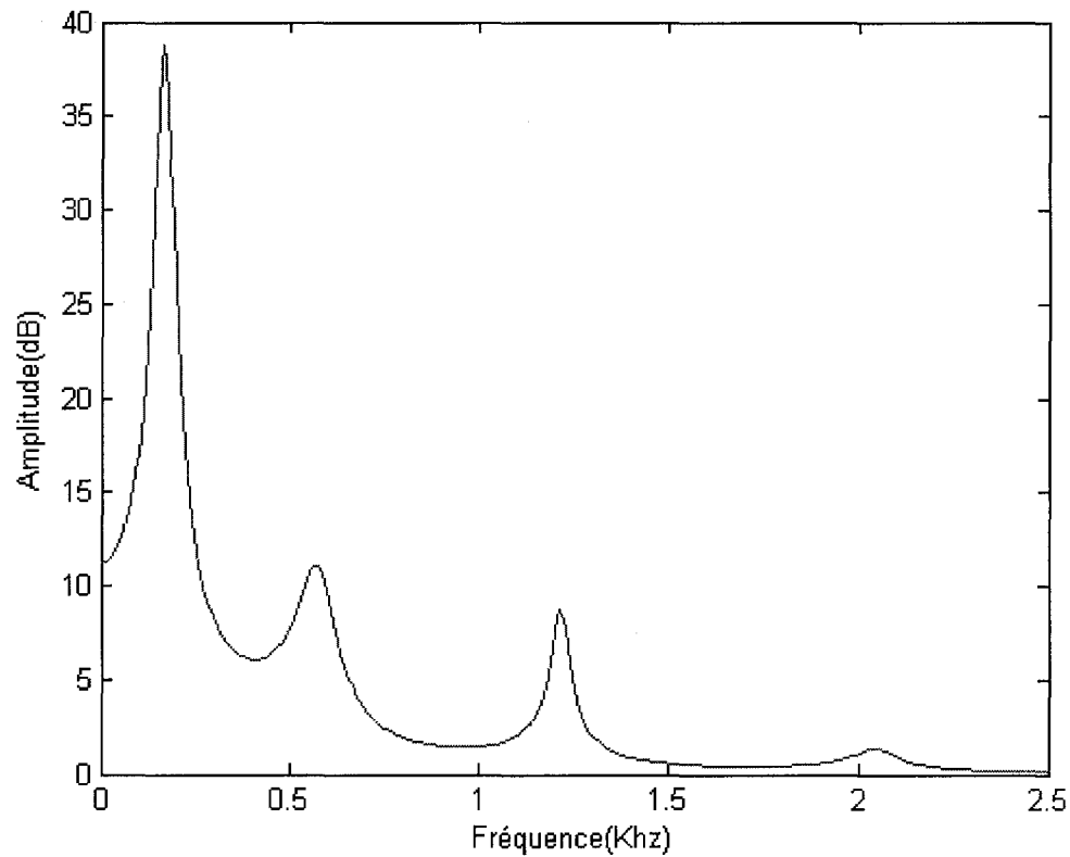
Figure 13 Exemple d'un spectre LPC
