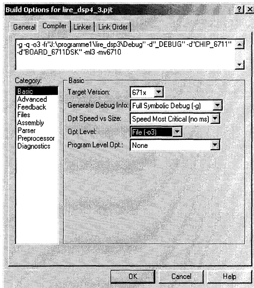
Figure 38 La configuration du projet
