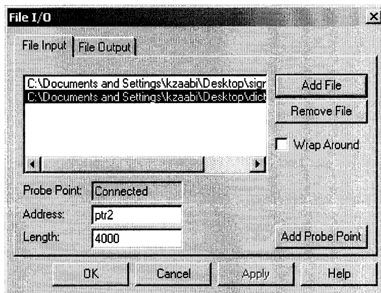
Figure 44 Lecture/Écriture des fichiers à l'aide de sondes
