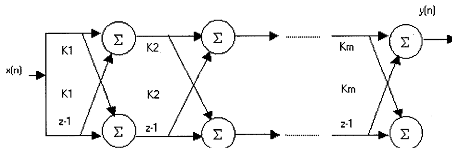
Figure 16 Structure en treillis d'un filtre
