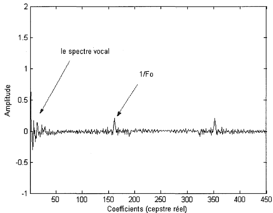
Figure 17 Exemple d'analyse homomorphique
