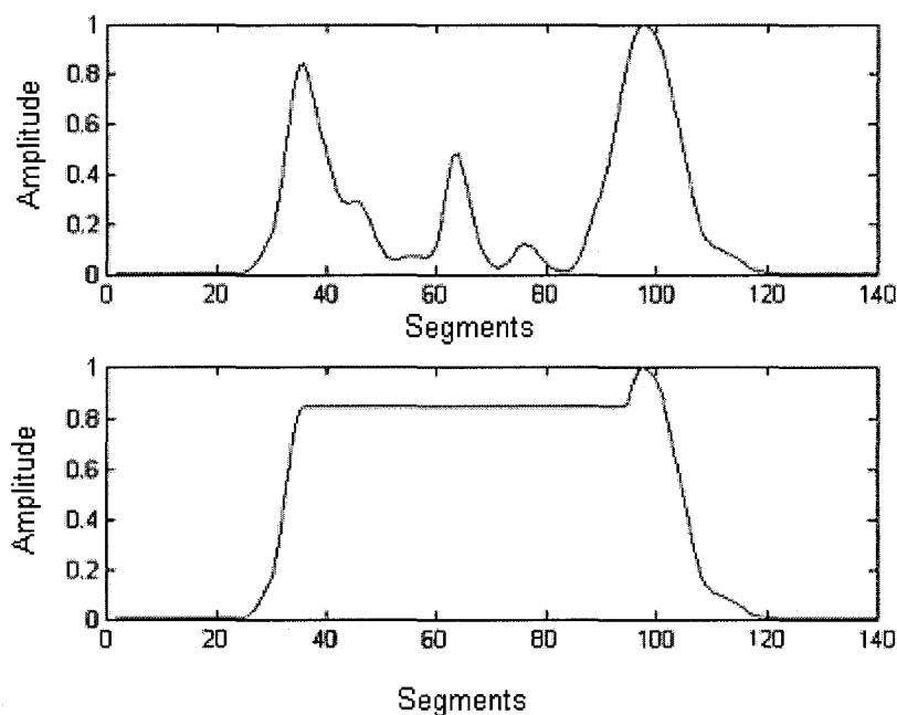
Figure 26 La fonction convexe-hull de l'énergie du signal
