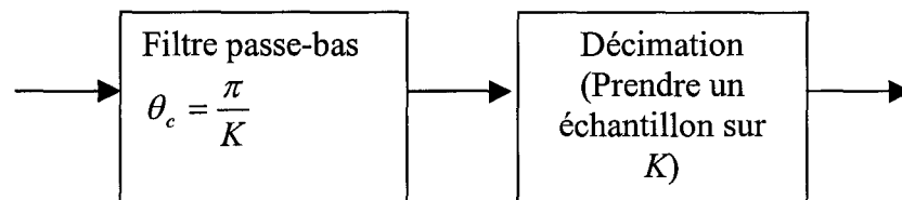
Figure 40 La décimation par un facteur K
