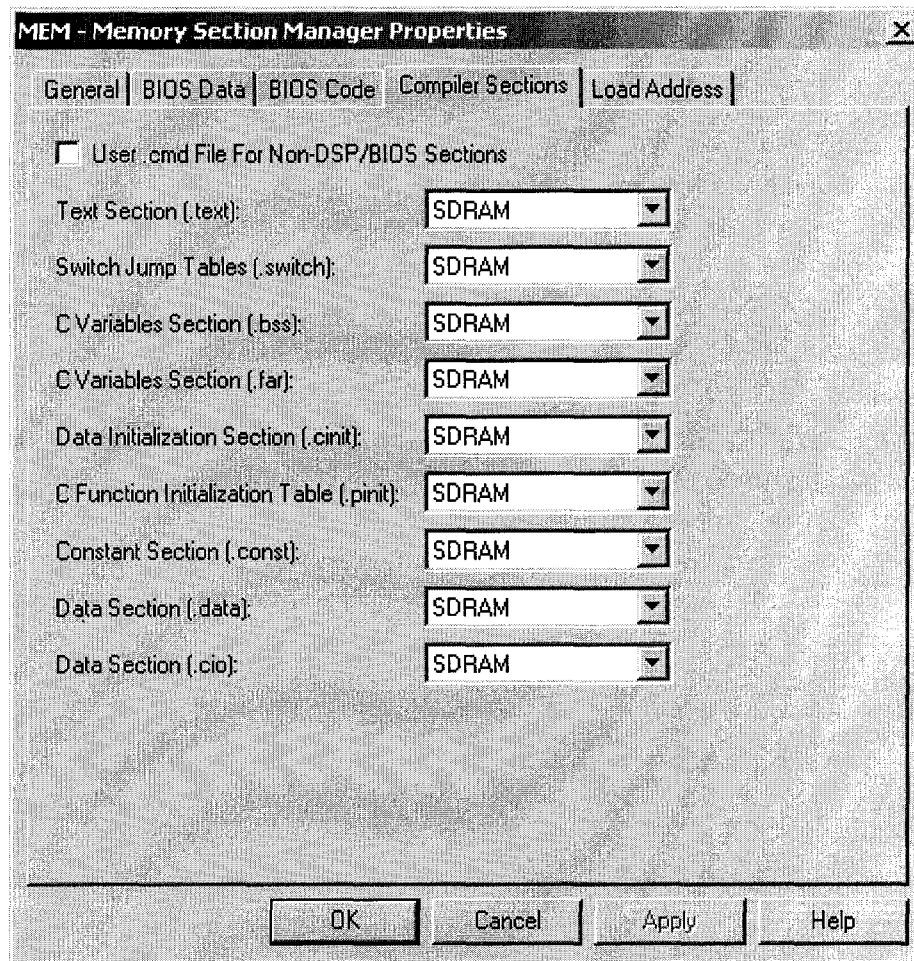
Figure 37 L'organisation de la mémoire via le gestionnaire de mémoire MEM
