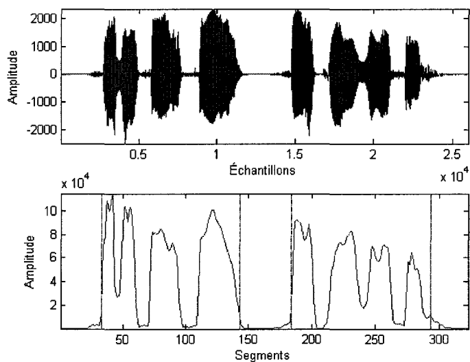
Figure 47 Suppression du silence à l'intérieur du signal
