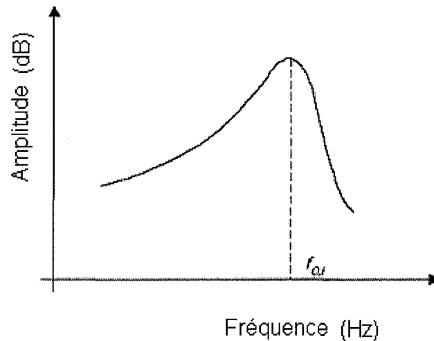
Figure 7 Réponse en fréquence d'une cellule ciliée [13]
