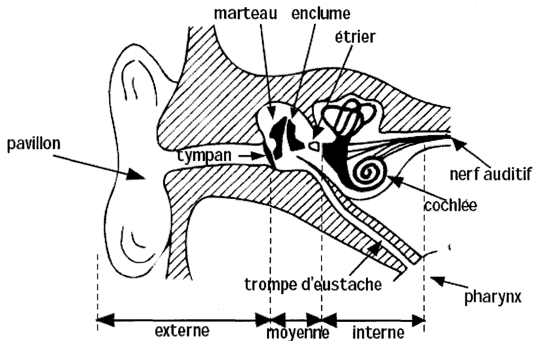
Figure 6 Structure du système auditif [13]
