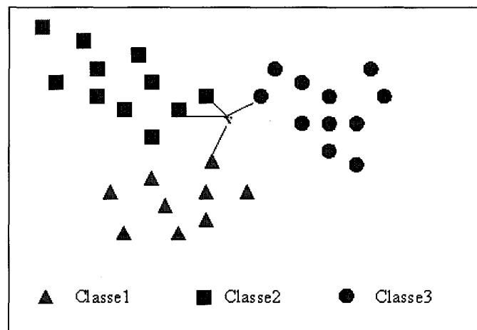
Figure 30 Principe du plus proche voisin : l'élément x est affecté à la classe2
