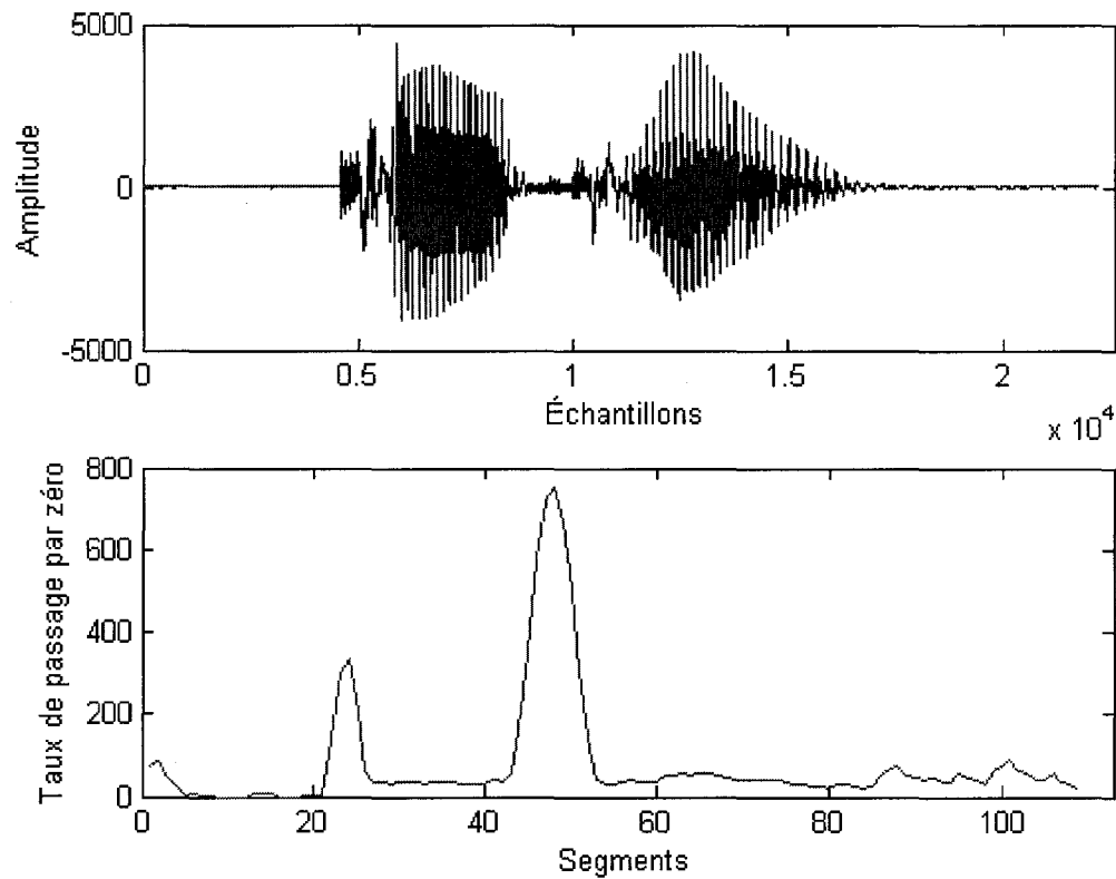
Figure 12 Le taux de passage par zéro d'un signal vocal
