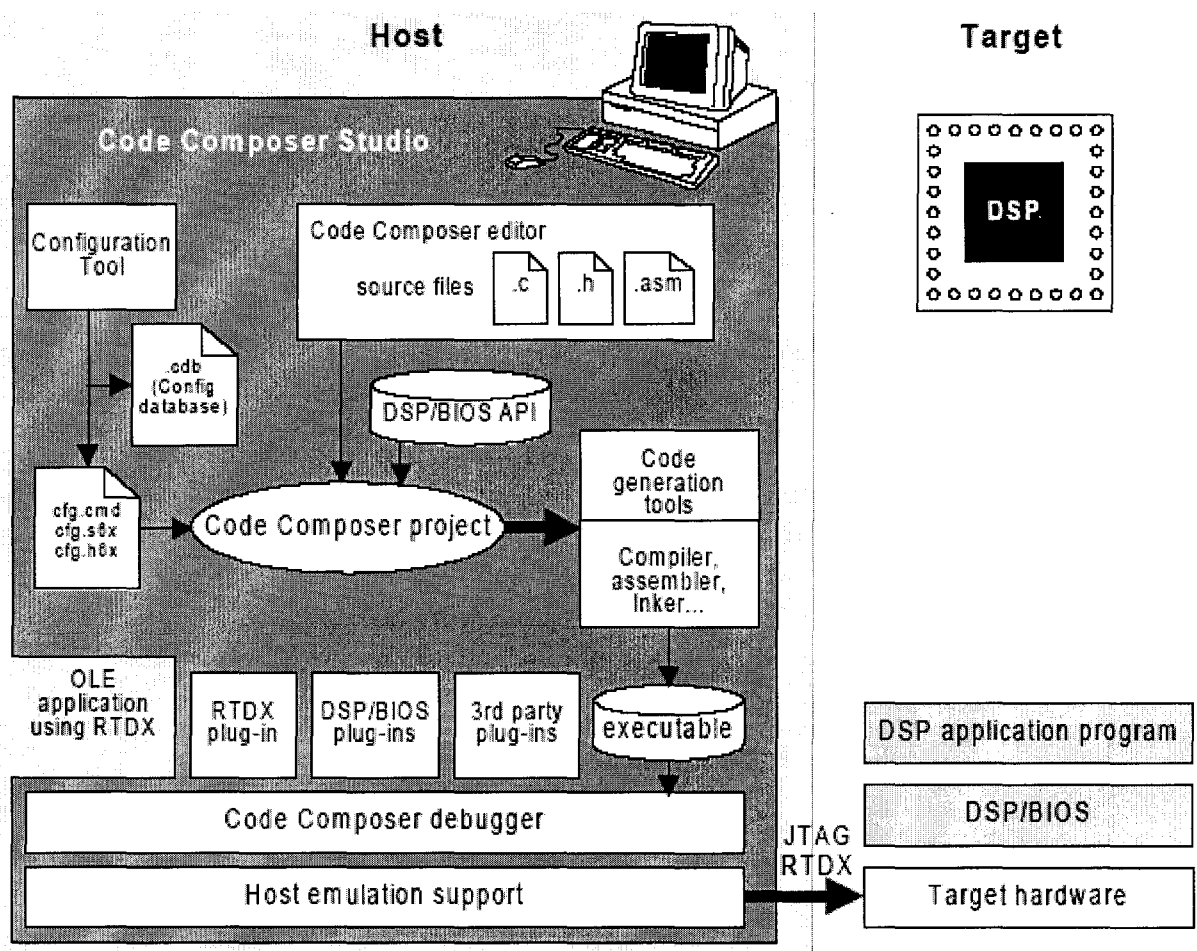
Figure 33 Structure du système du développement du TMS320C6711 [57]
