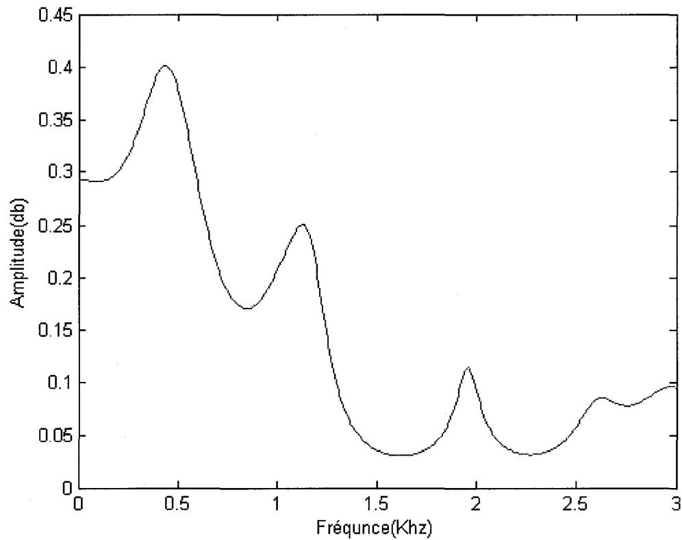
Figure 18 Lissage cepstral obtenu avec des coefficients LPCCs
