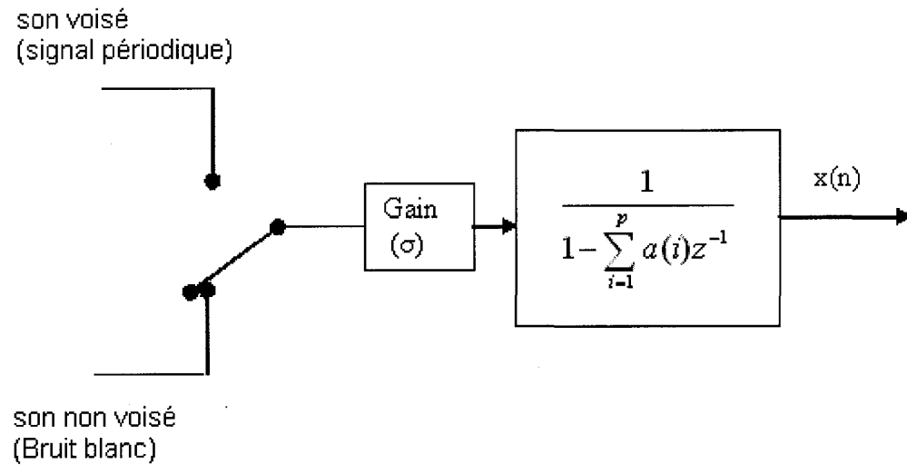
Figure 15 Modèle auto régressif
