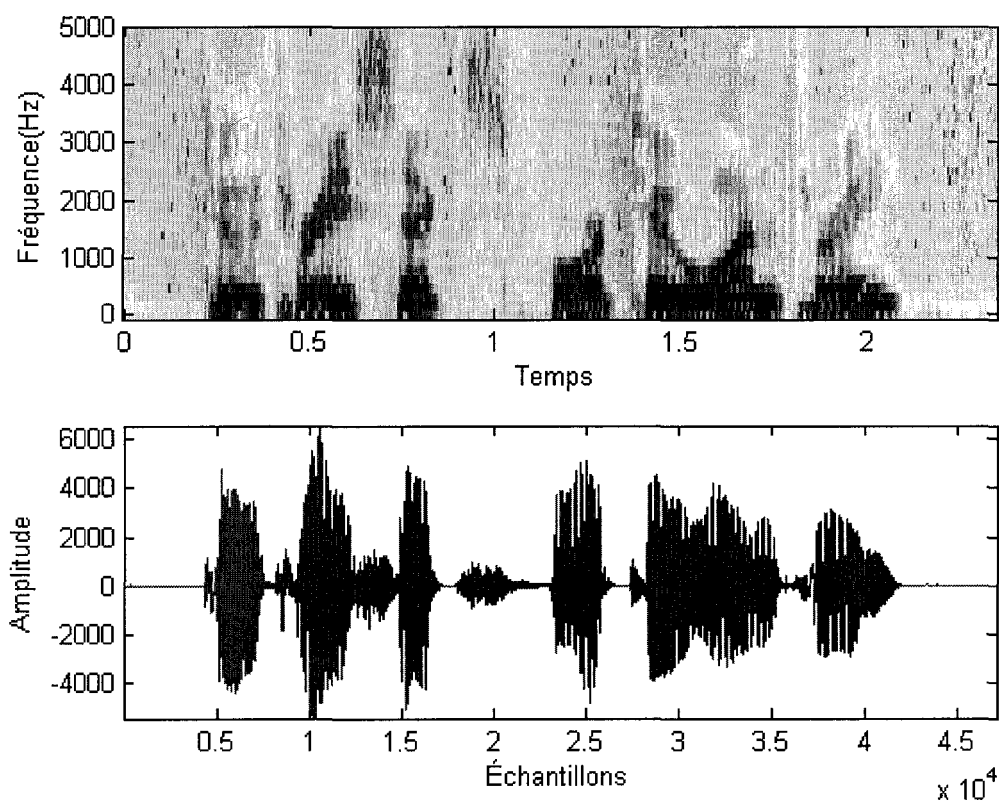
Figure 4 Spectrogramme à bande large (128 échantillons)
