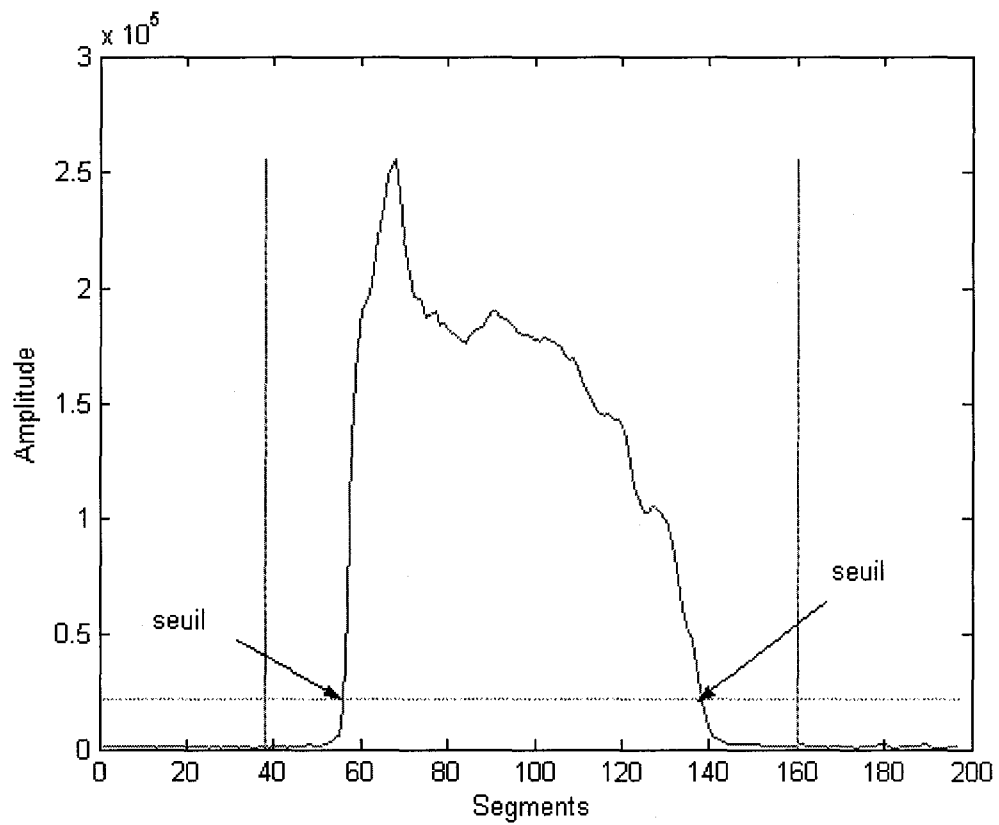
Figure 29 Sélection de la partie énergétique du signal à l'aide d'un seuil
