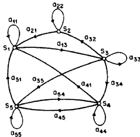
Figure 21 Modèle de Markov à 5 états [3]
