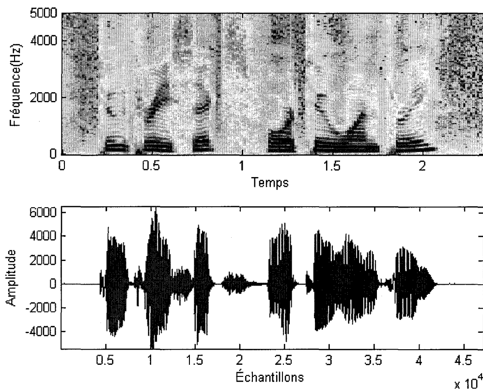
Figure 5 Spectrogramme à bande étroite (512 échantillons)
