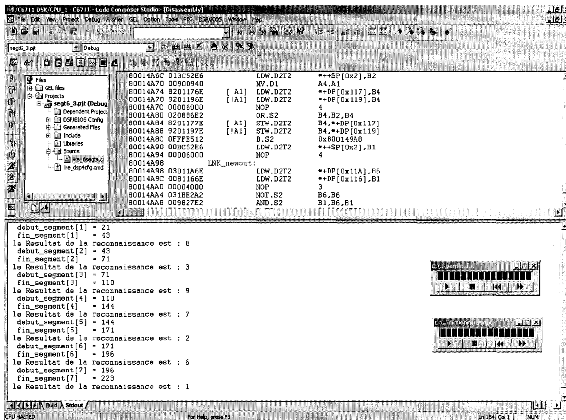
Figure 45 Affichage du résultat de reconnaissance après traitement
