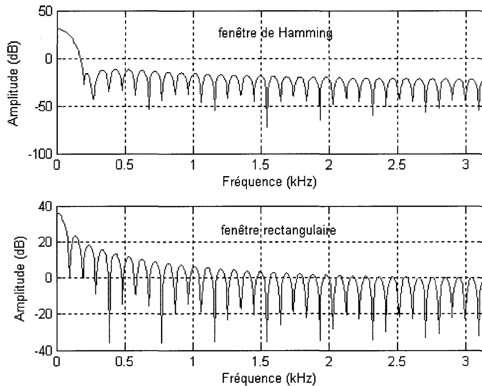
Figure 10 Spectre des fenêtres de Hamming et Rectangulaire
