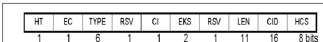
Figure 1.9 En-tête MAC générique.
