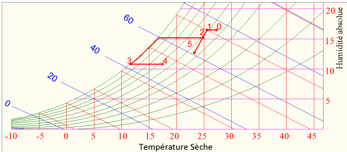
Évolution de l'air sur le diagramme psychrométrique pour la région A
