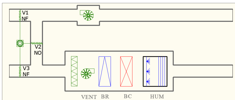
Figure 1.6 Système à débit d'air constant
