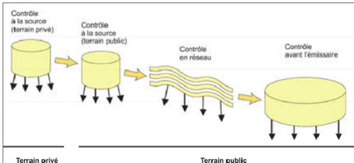
Figure 2.4 Catégorisation des PGO en fonction de leur localisation dans le réseau de drainage
