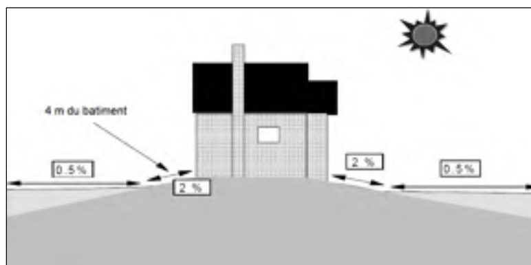
Figure 2.5 Pentés des terrains (adapté de MOE 2003) Adaptée du MOE (2003, p. 4-16)
