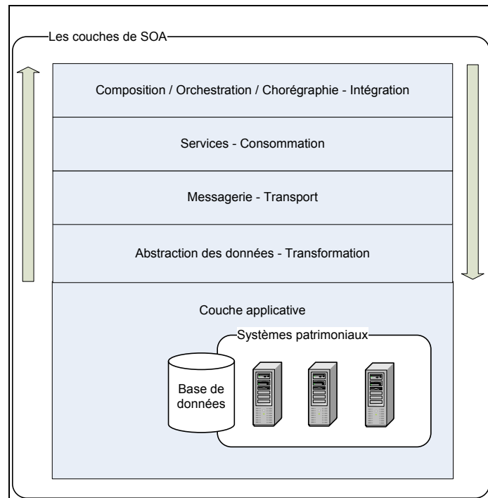
Figure 1.2 Les couches d'une SOA. Adaptée de (Arsanjani, 2004)
