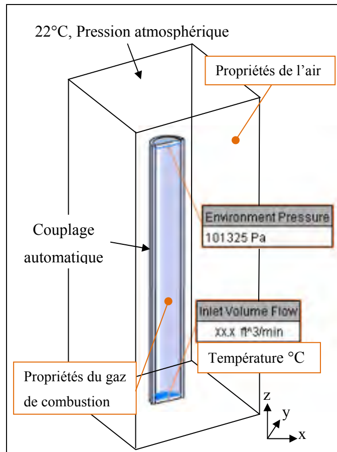
Figure 3-3 Modèle de la conduite verticale cylindrique
