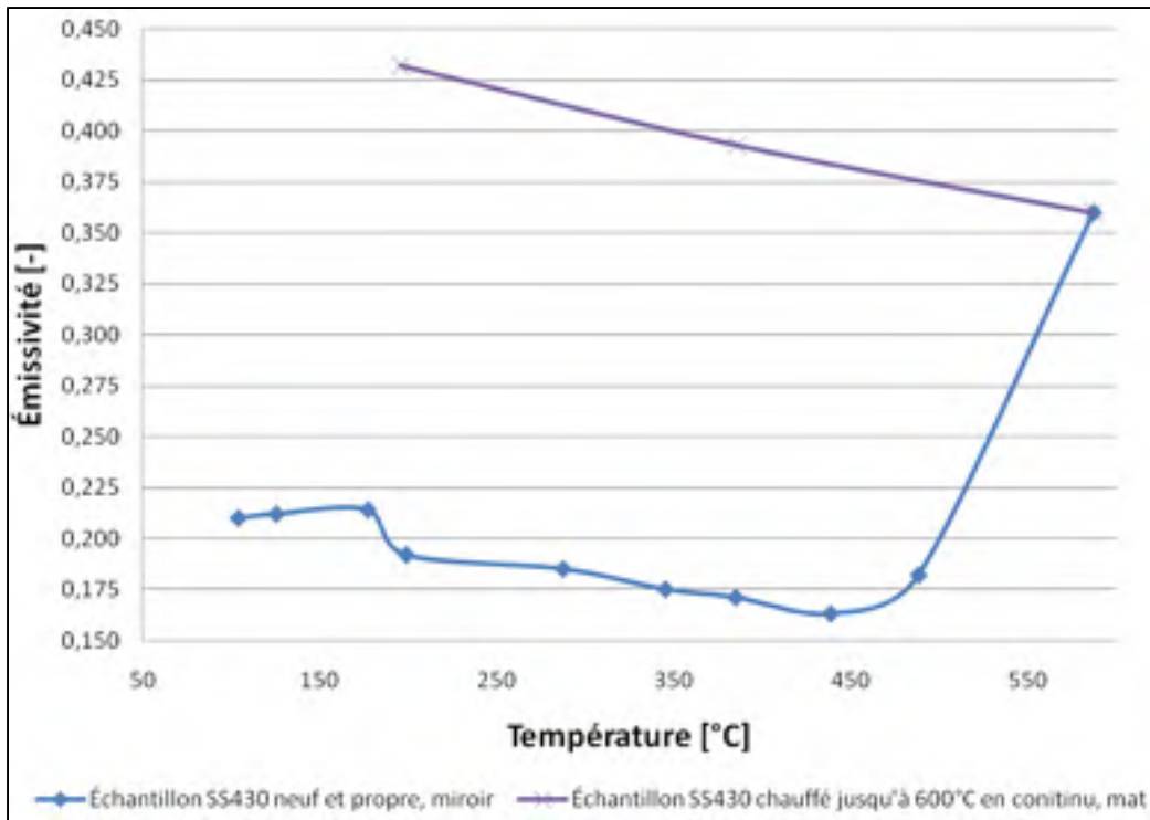
Figure 2-11 Émissivité de l'acier inoxydable 430
