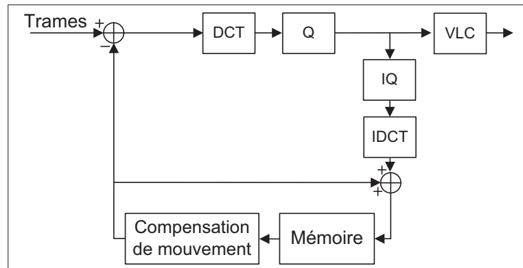
Figure 1.1 Schéma de principe d'un codeur vidéo.
