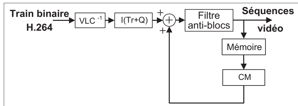
Figure 1.10 Décodeur H.264.
