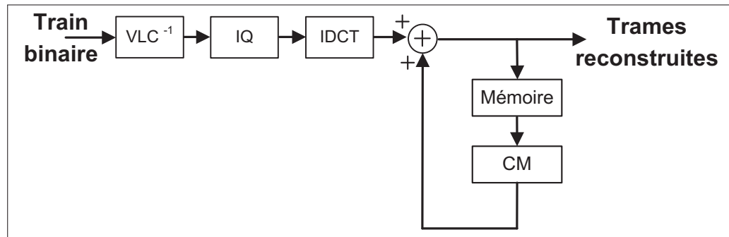
Figure 1.6 Schéma de principe d'un décodeur vidéo.
