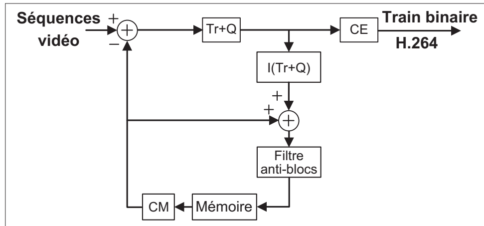
Figure 1.9 Codeur H.264.
