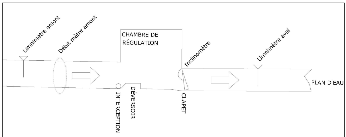
Figure 2.1 Emplacement des instruments dans un émissaire de débordement
