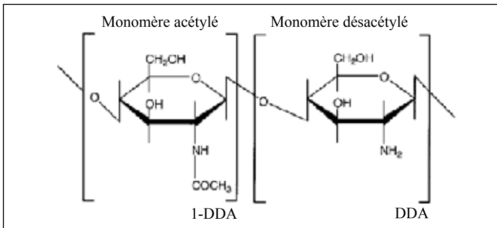
Figure 1.10 Les deux monomères composant le chitosane Adaptée de Desbrieres (2002)
