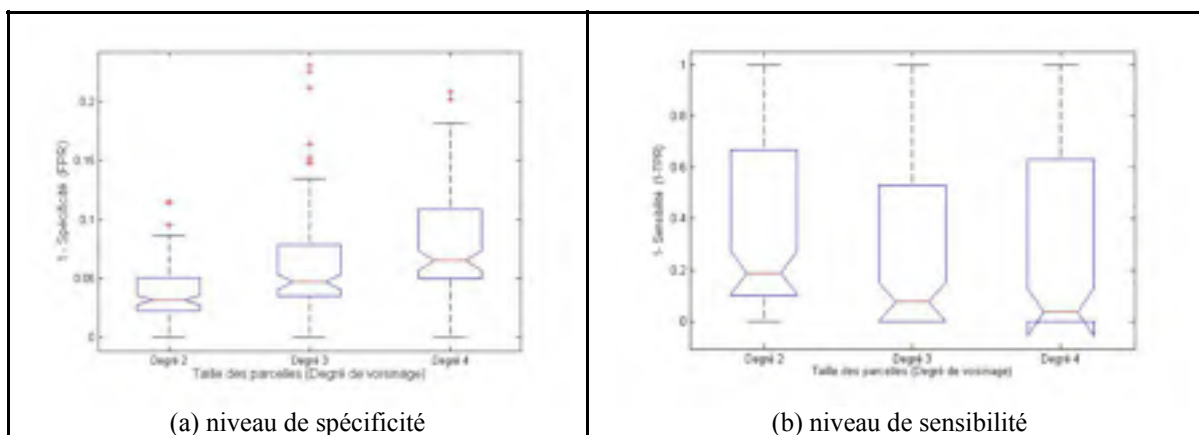
Figure 5.14 Analyse ROC de la localisation des sources avec une tolérance FP de 1% et des données avec un rapport signal/bruit de 10^{-4}
